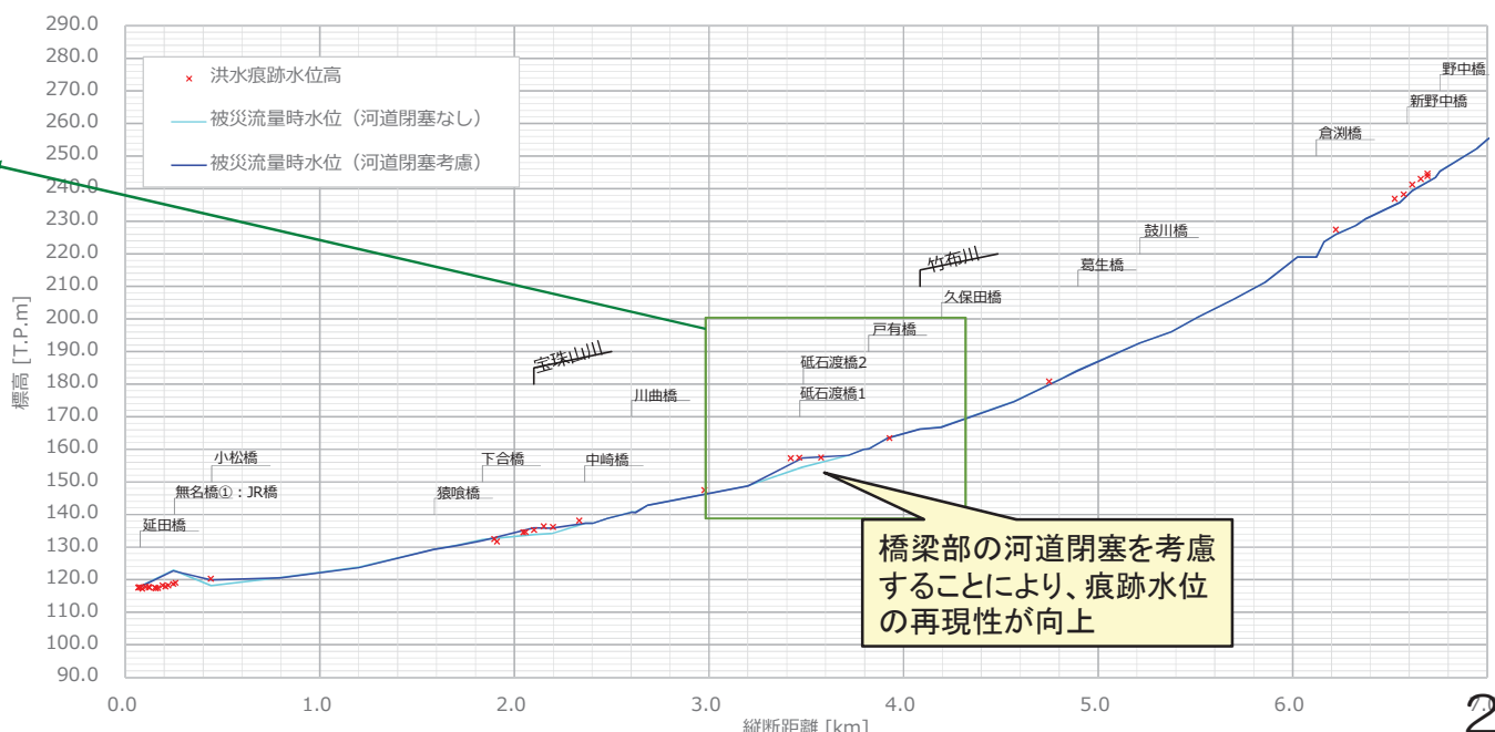
洪水痕跡水位計算結果 (大肥川0k070~7k000)
