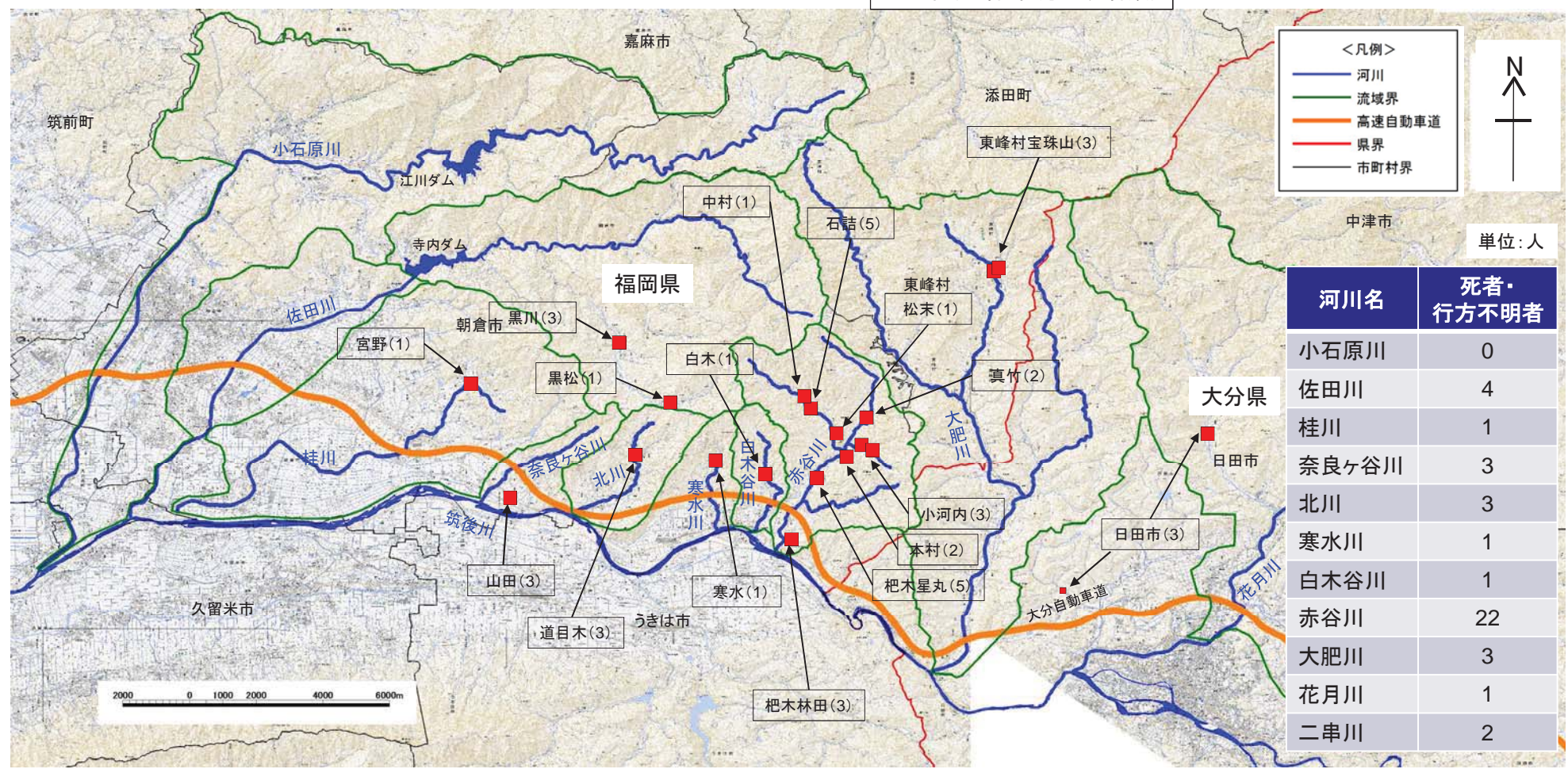
死者・行方不明者の推定発生箇所
