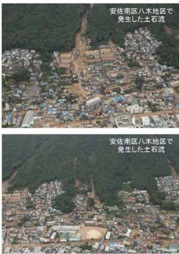
※出典:2014年8月広島大規模土砂災害緊急調査 報告書 平成27年3月 砂防学会他
