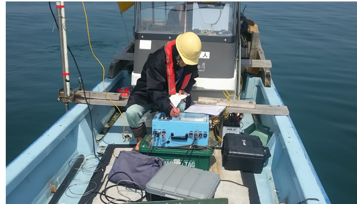
▲音響測深機による深浅測量を実施。
