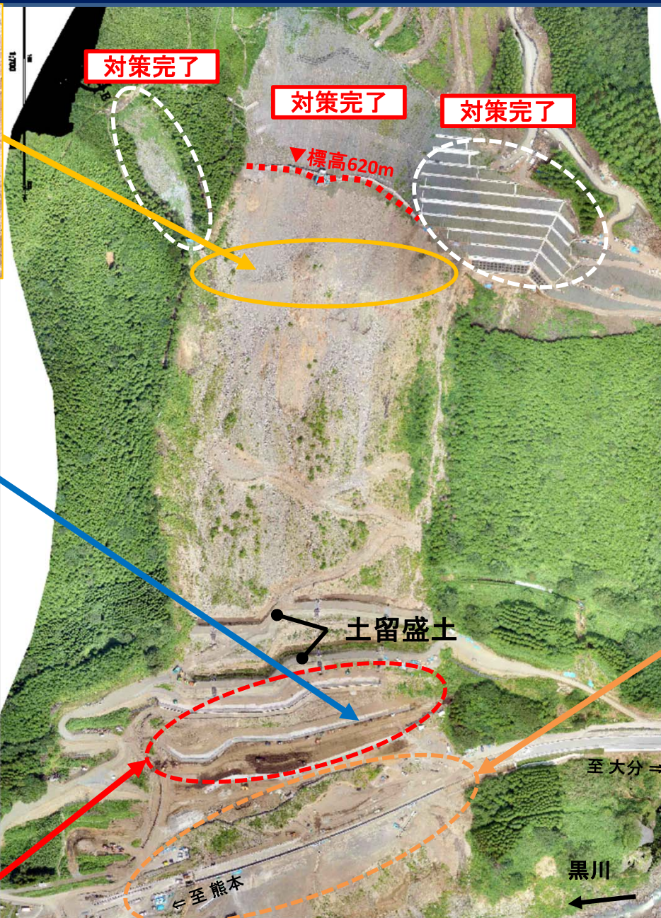
斜面上部~中腹部: 傾斜の特に急な標高620m付近まで対策完了 崩壊土砂の撤去標高540m付近施工中
