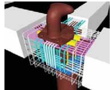
【CIMモデルの活用事例】
