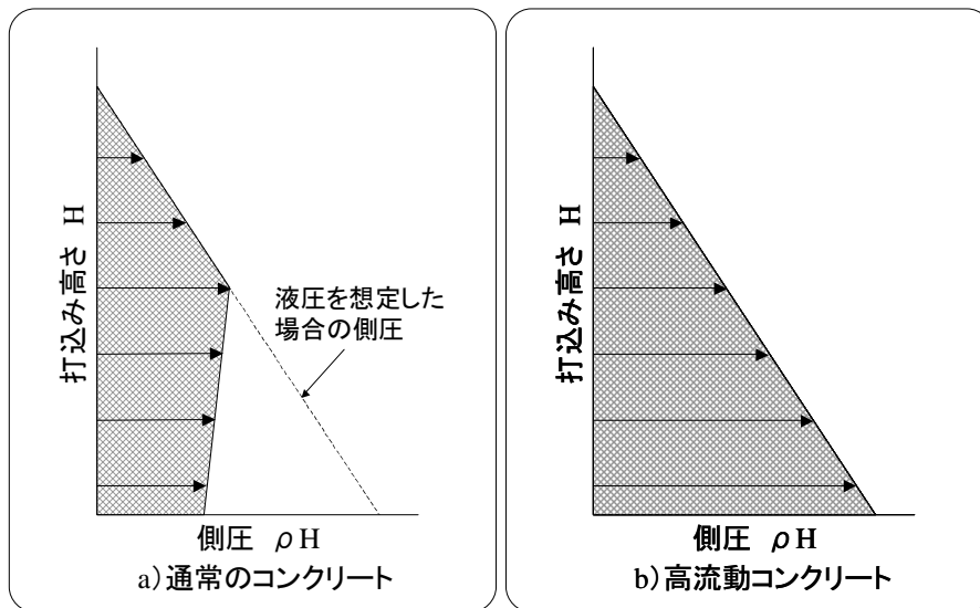
解説 図 3.12.1 型枠に作用する側圧
