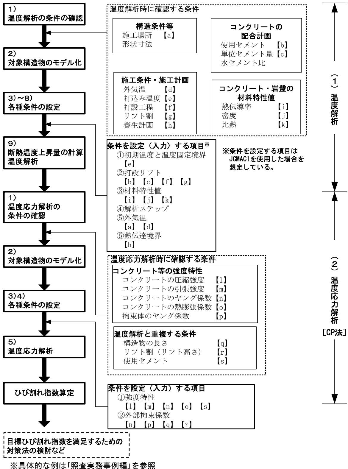
図 3.5.1 温度応力解析フロー（CP法：JCMAC1の例）
