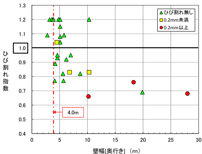
図 3.3.4 施工実態調査に基づく温度応力解析結果とひび割れ発生状況(壁)
