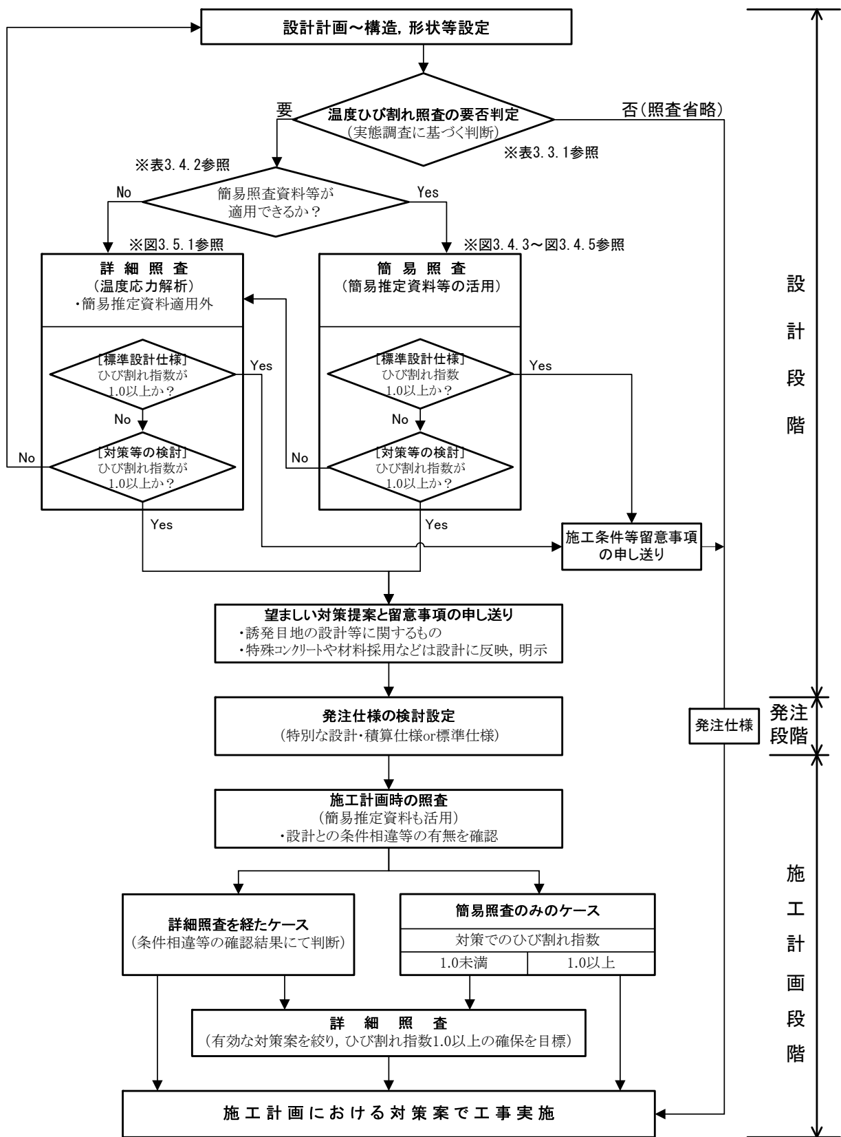
図 3.2.1 温度ひび割れ照査フロー
