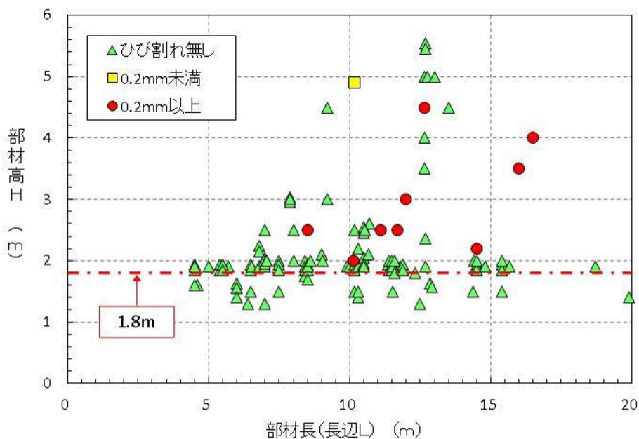
図 3.3.1 ひび割れ発生状況と緩和対象ライン（フーチング）
