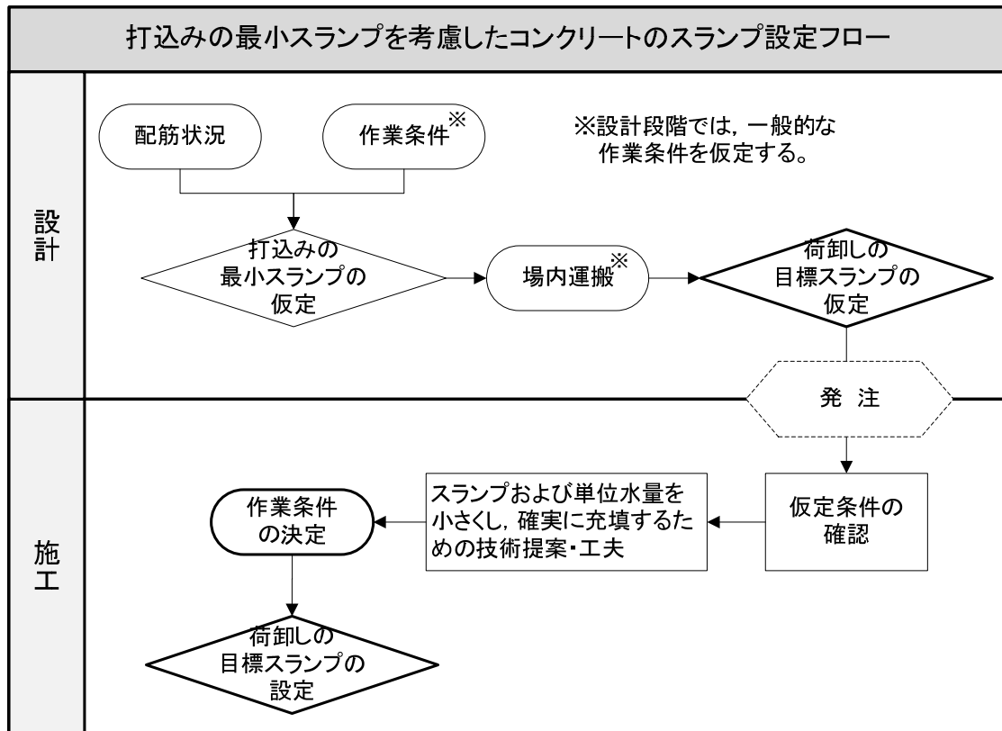
図 2.1 打込みの最小スランプを考慮したスランプ設定フロー
