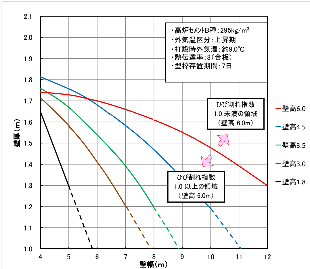
図 3.4.4 壁(柱)部材：ひび割れ指数 1.0 の境界図[例]
