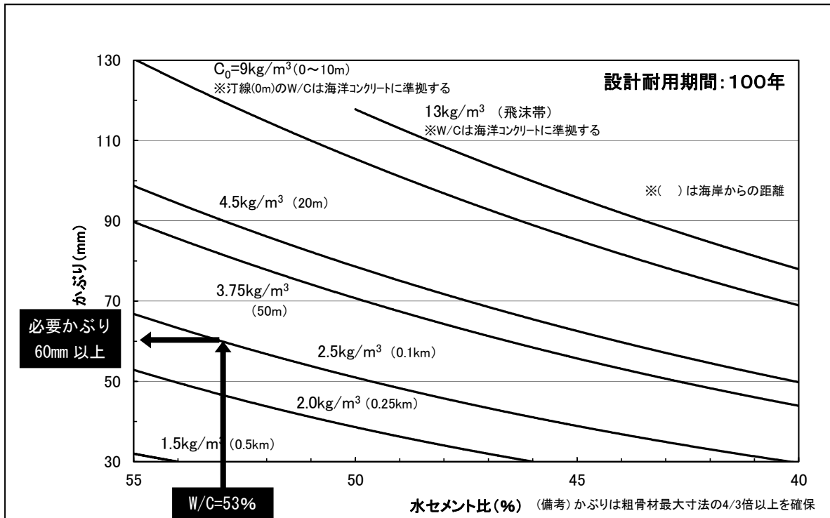
図 1.3 塩害に対する照査を満足する水セメント比およびかぶり判定図
