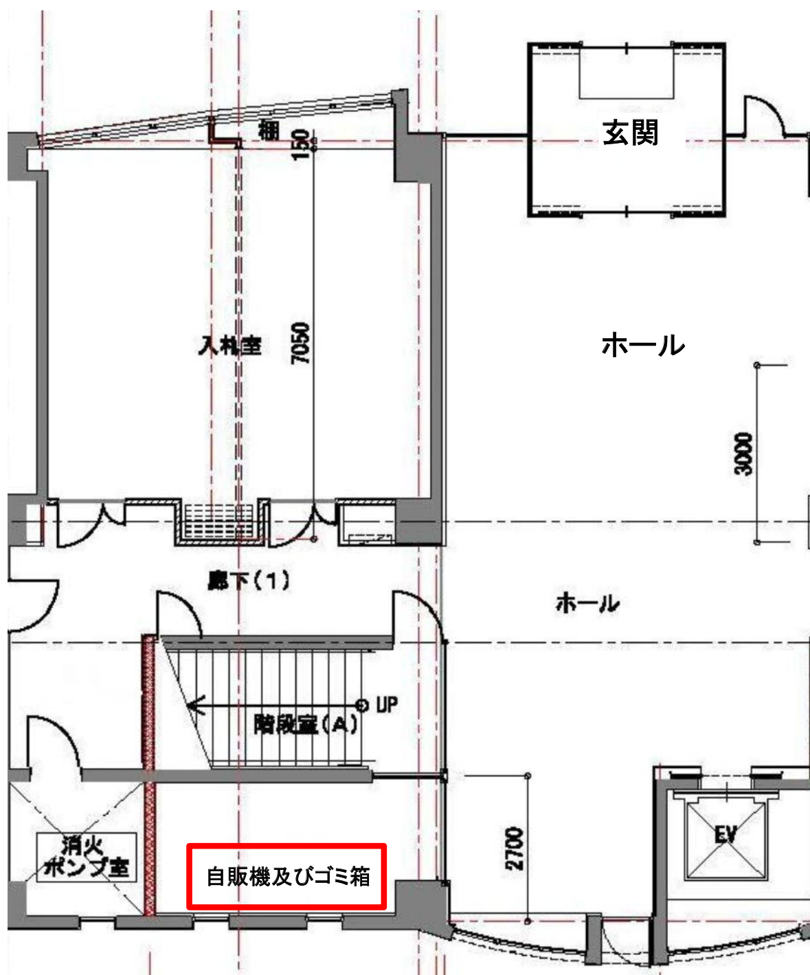
配置図
