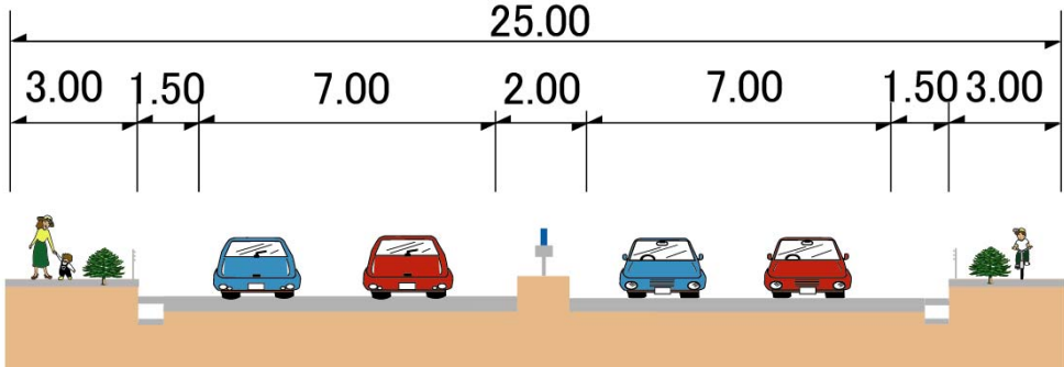
▲標準横断面(単位:m)
