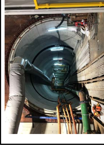
(シールド工事施工状況)
