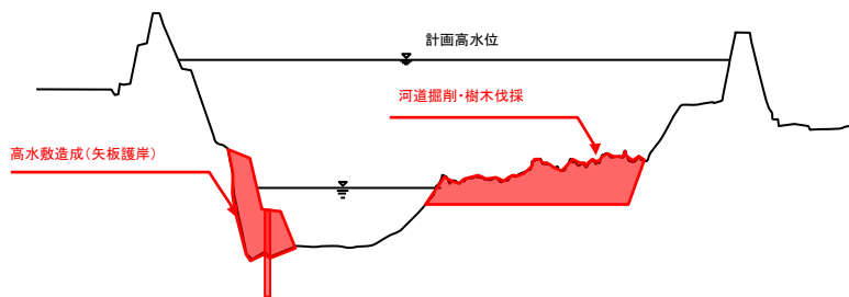
標準断面図
