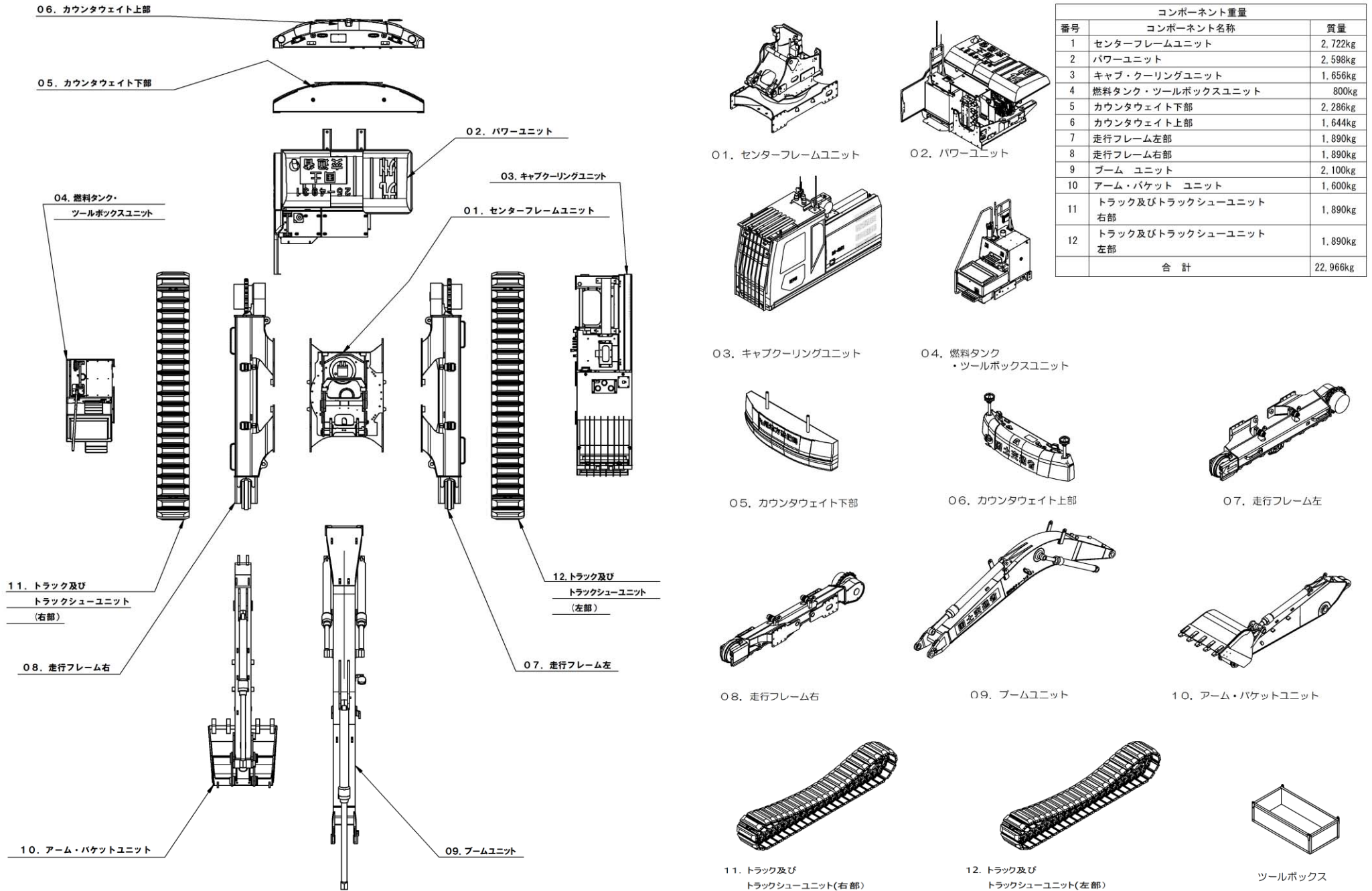
分解型BH分解図
