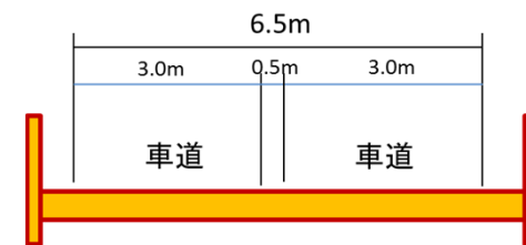
仮橋横断面図
