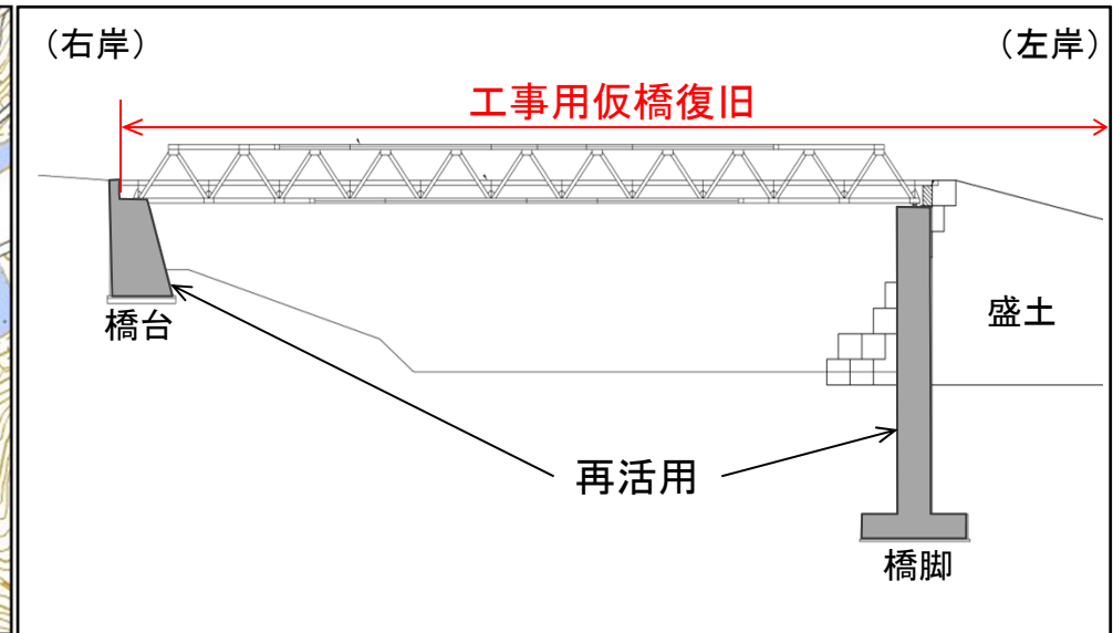
工事用仮橋の復旧図
