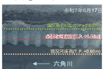
写真②(洗掘状況)
