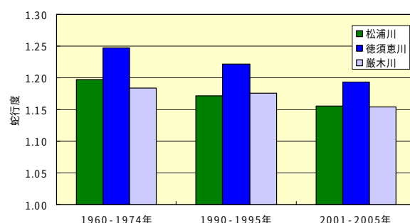
図 2.3.9 蛇行度の変化
