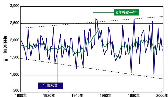
図 2.2.5 佐賀の年降水量の経年変化
