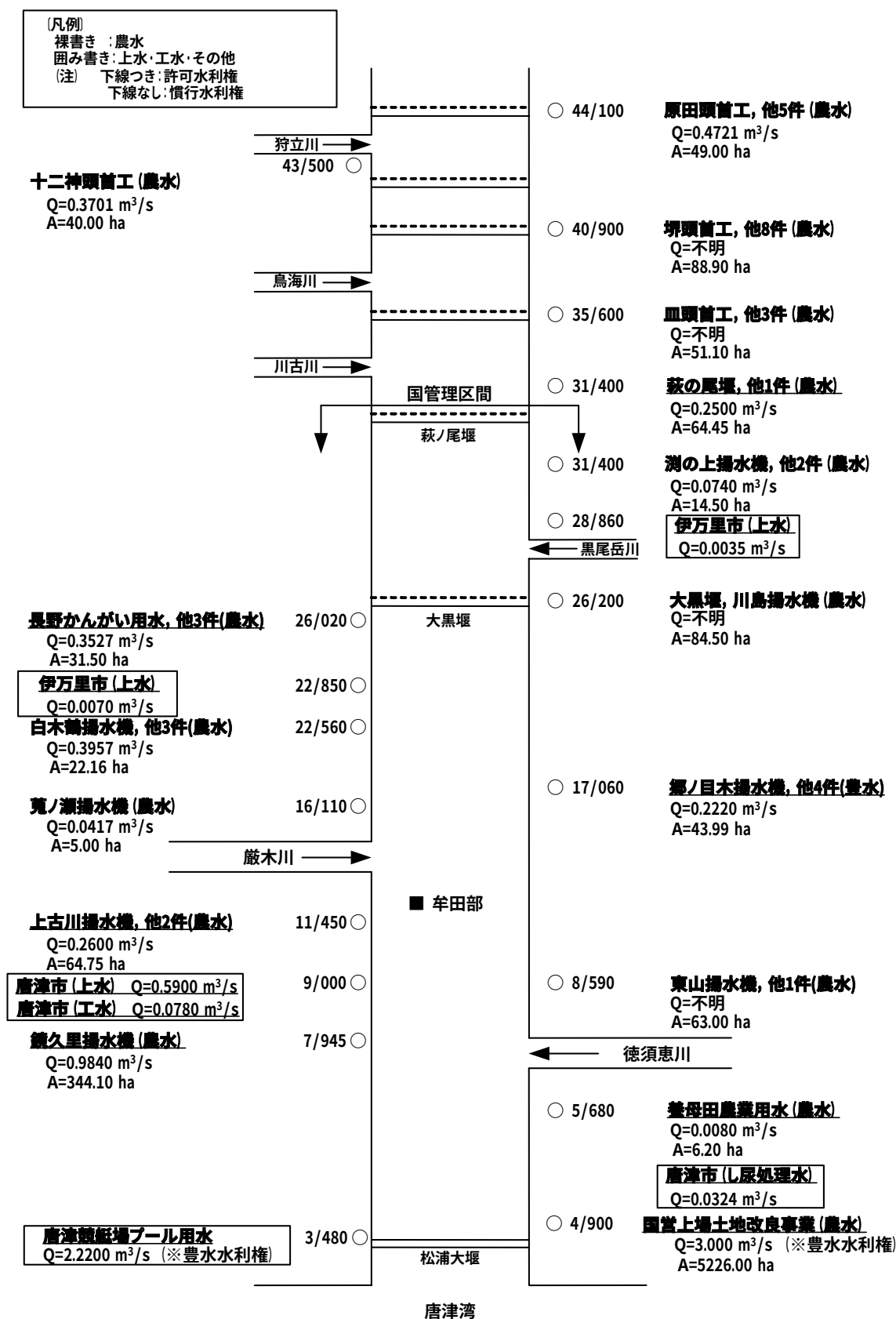
図 2.2.2 松浦川水系の主な水利用の現況模式図
