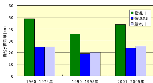
図 2.3.8 自然水際距離の変化
