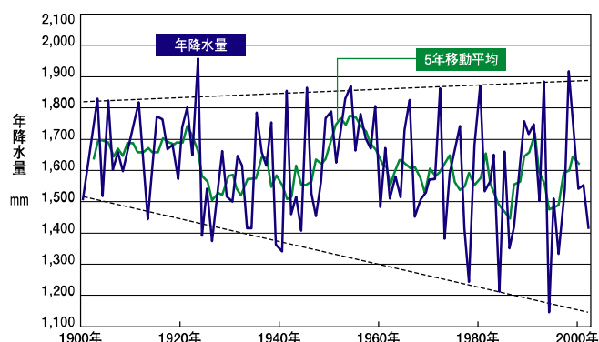
図 2.2.4 日本の年降水量の経年変化
