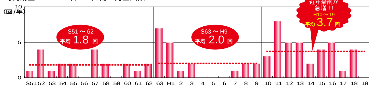
図 2.1.7 時間雨量 50mm、100mm 以上の降雨発生回数
