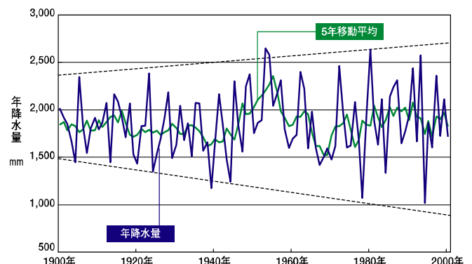
図 2.2.5 佐賀の年降水量の経年変化
