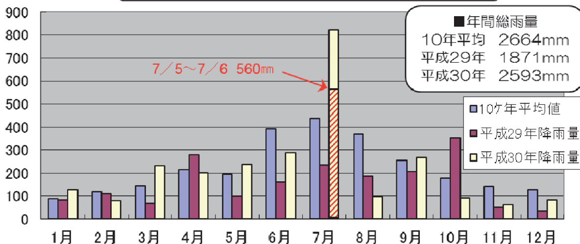
厳木ダム上流の流域平均雨量（平成30年）
