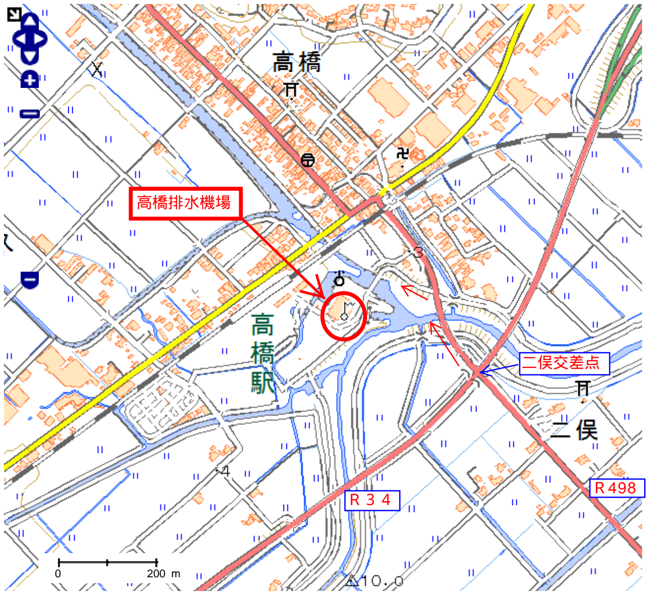
高橋排水機場 位置図
