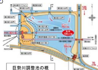
巨勢川調整池の概
