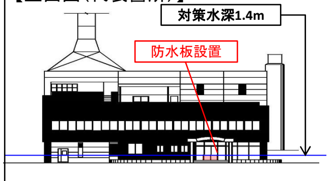
【立面図(代表箇所)】
