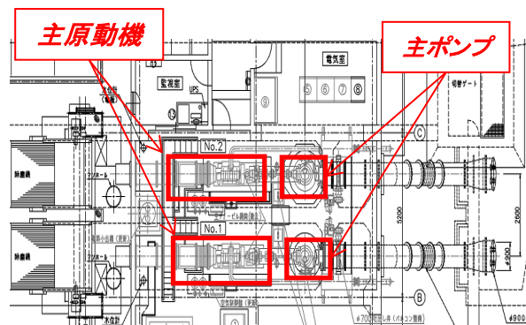
機場平面図
