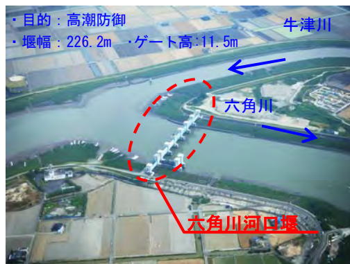
写真 1.2.21 六角川河口堰 (昭和 58 年 3 月完成)
