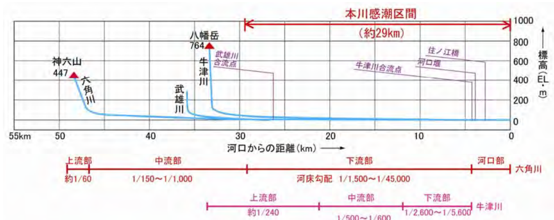
図 1.1.3 六角川本支川縦断面図
