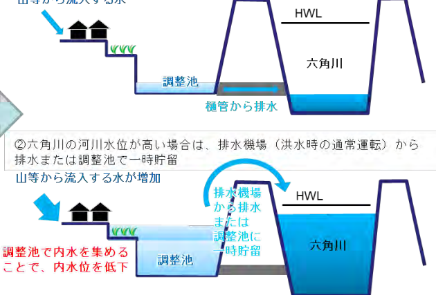
図-5.2 調整池による貯留イメージ
