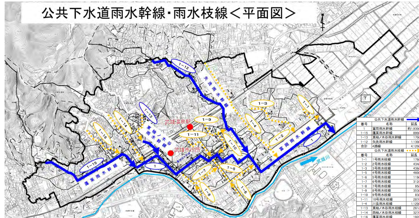
下水道の排水先の状況（富岡雨水幹線）
