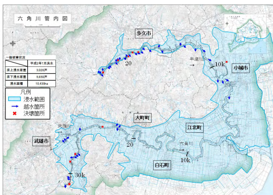
図-1.12 平成2年7月洪水での浸水区域
