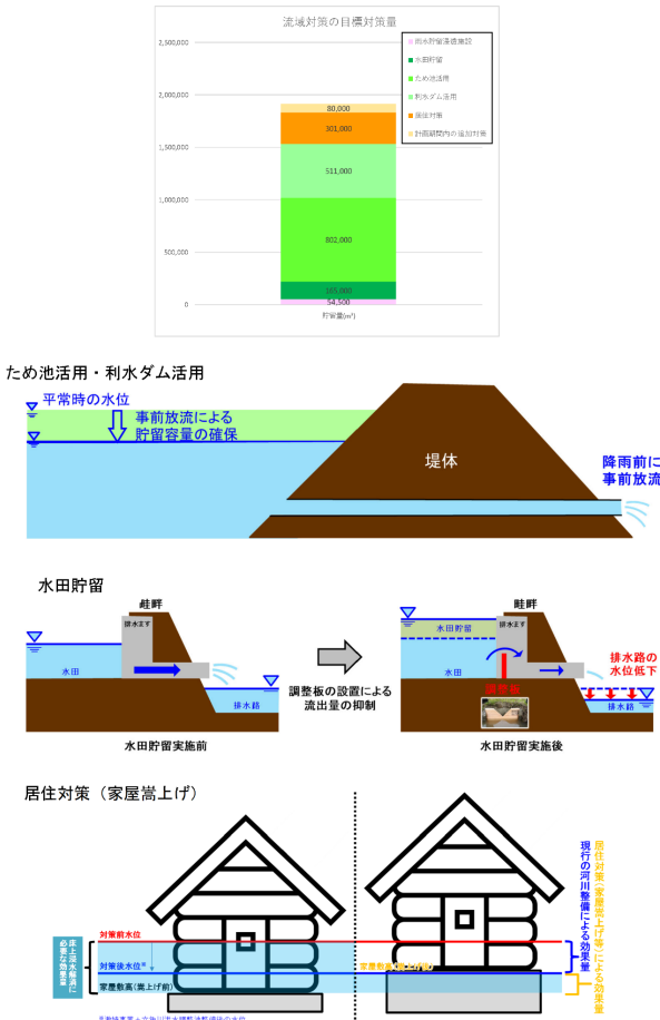
図-2.4 流域対策の目標対策量
