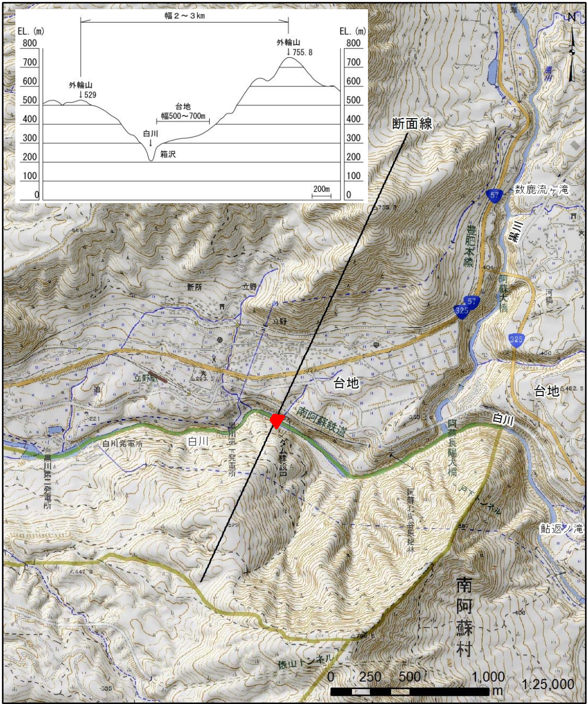
図-2.2.1 立野火口瀬周辺の地形と代表的な断面 (この背景地図等データは、国土地理院の電子国土 Web システムから提供されたものである。)
