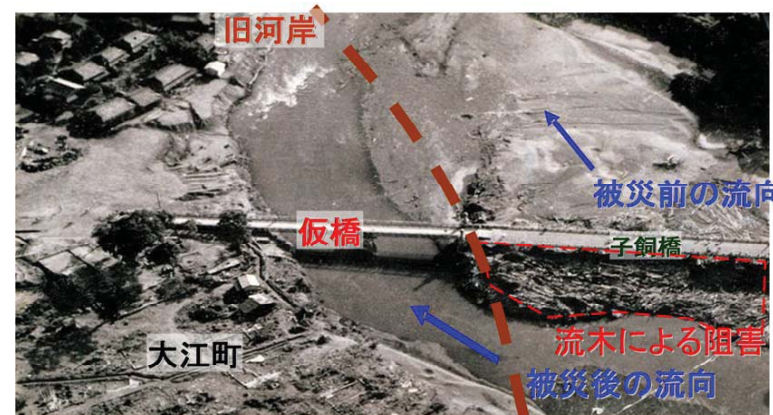
写真- 1.2.3 洪水後の子飼橋付近の状況
