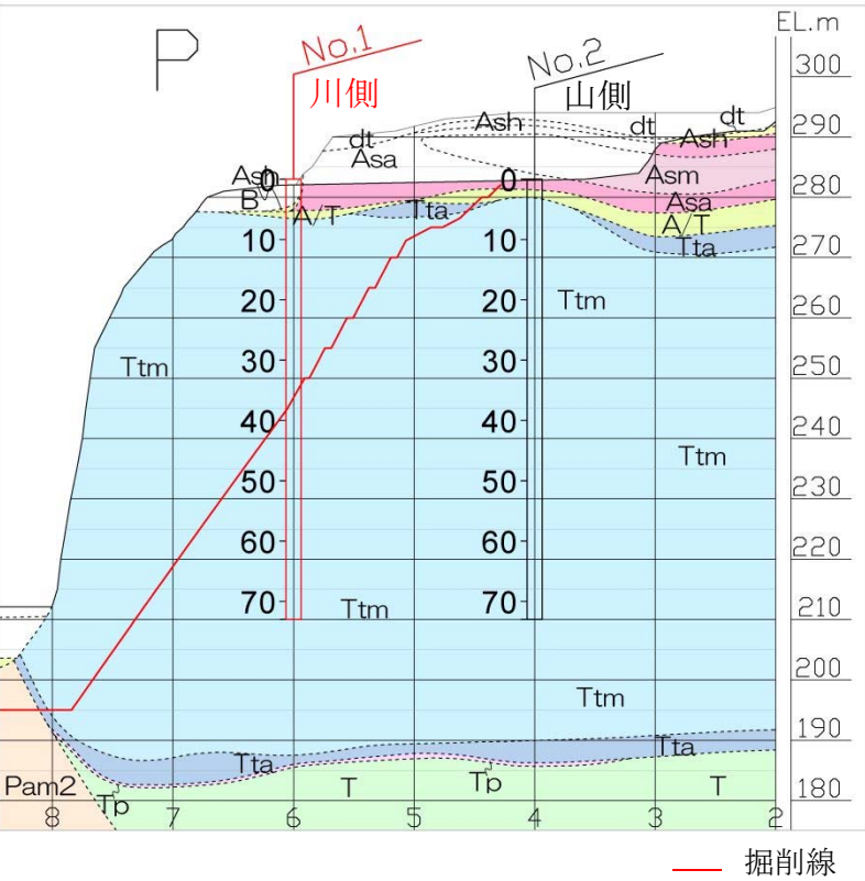
図-4. 3. 4 ボーリング横断図
