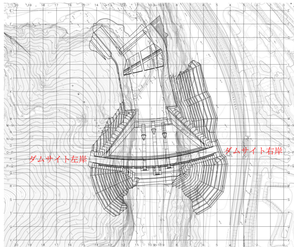
図-4.3.3 立野ダム平面図
