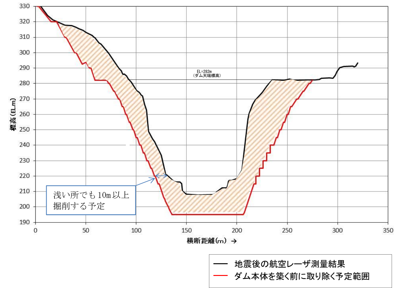
図-4.2.4 基礎掘削断面図
