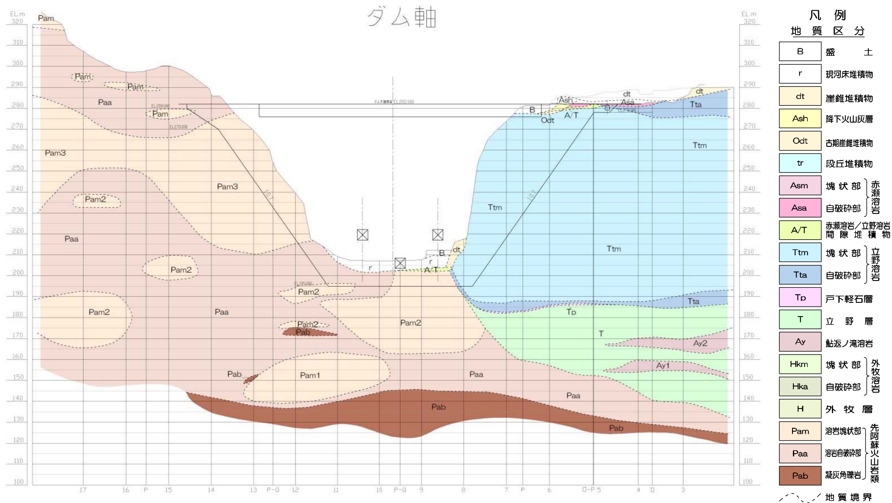
図-4.1.4 ダム軸の地質断面図
