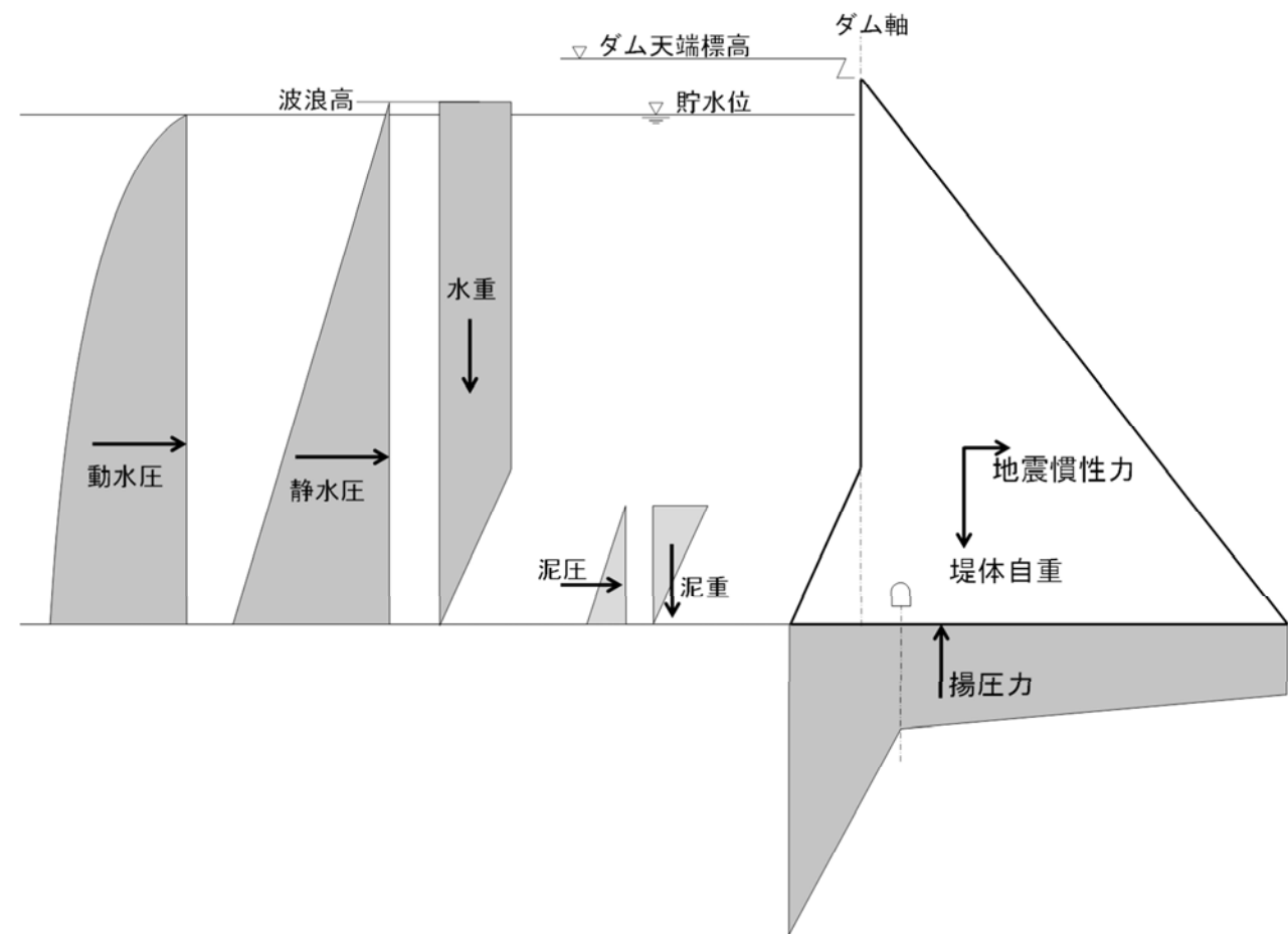
図-4.2.3 荷重条件の模式図
