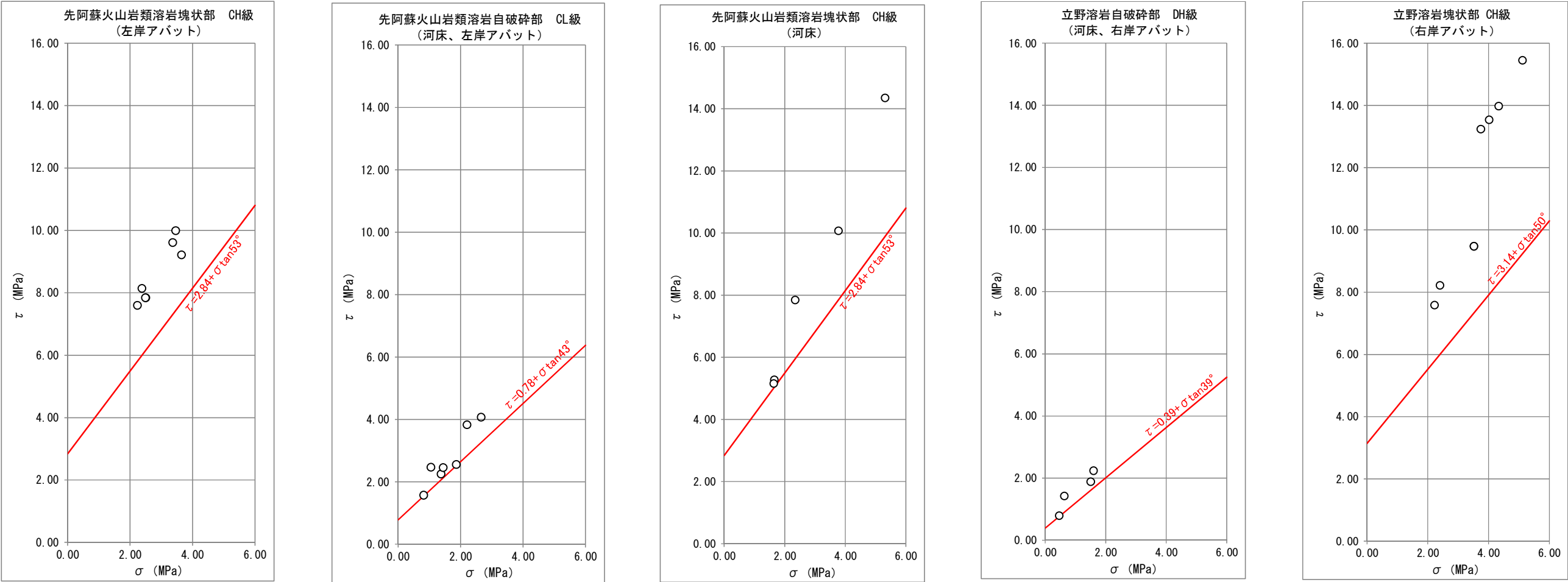
図-4.2.2 原位置せん断試験結果
