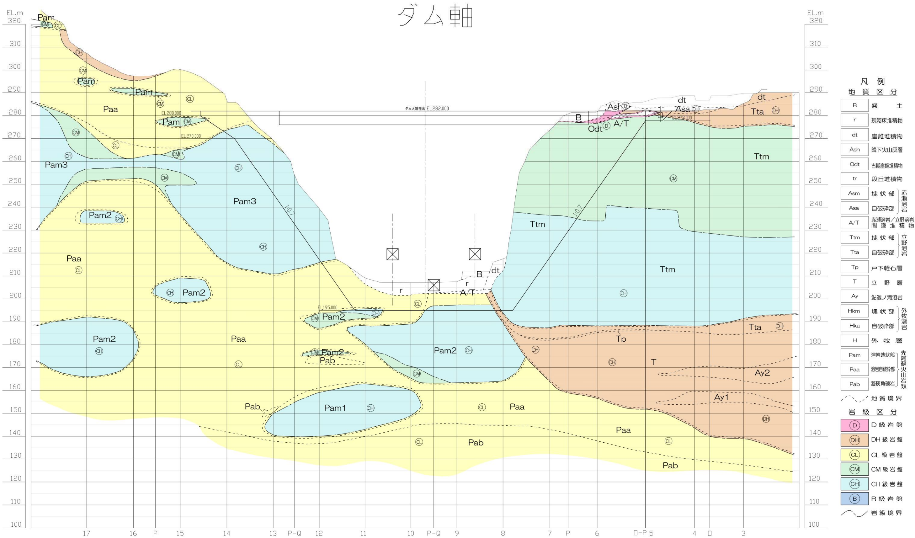
図-4.2.1 ダム軸の岩級区分図
