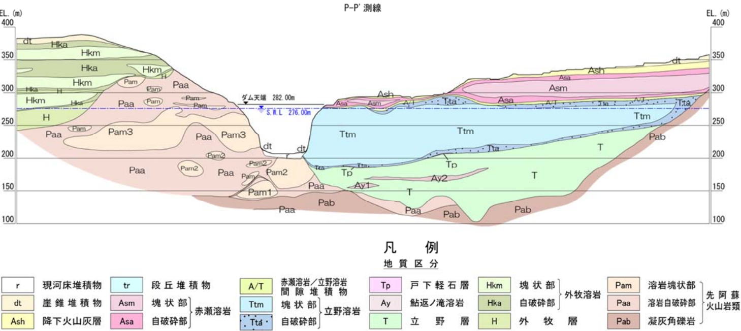
図-4.1.1 ダムサイト周辺の模式地質断面図
