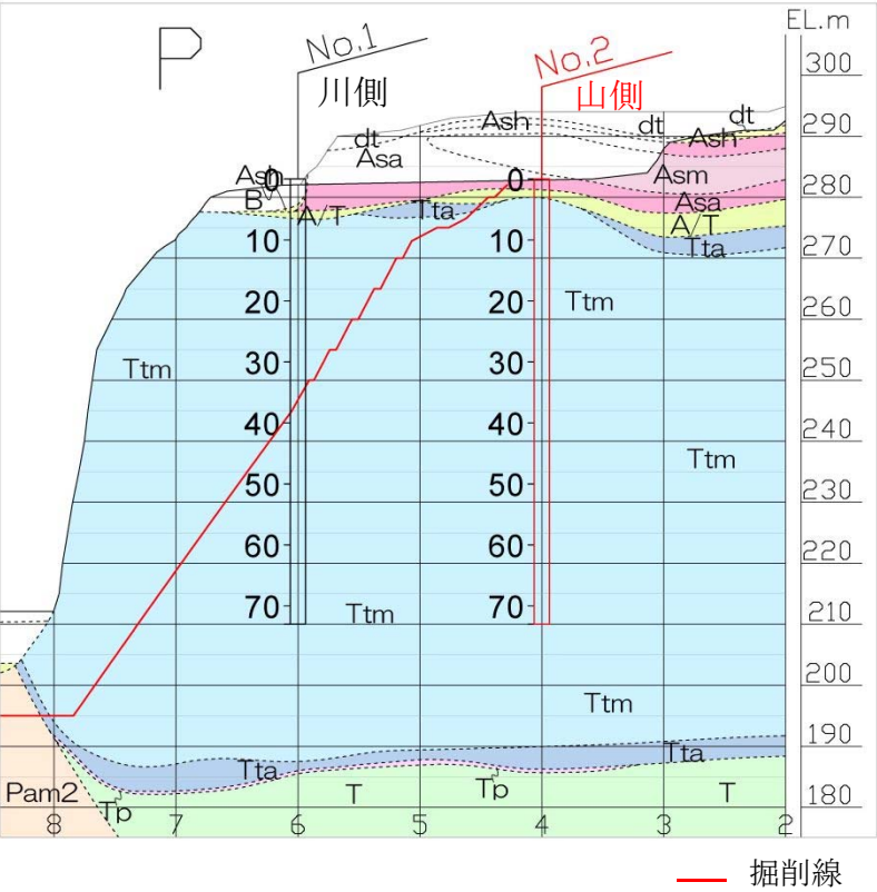
図-4.3.7 ボーリング横断図
