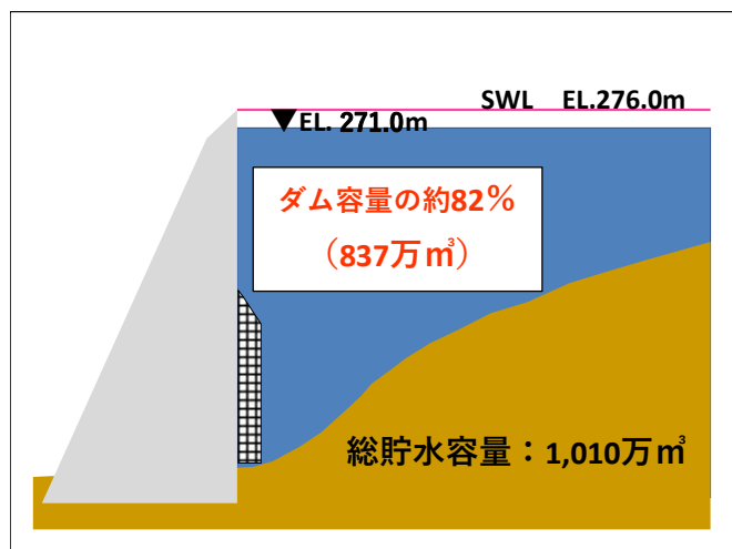
貯水容量イメージ
