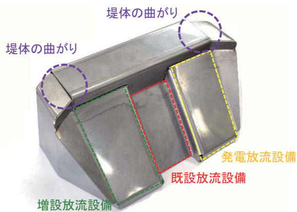
ご飯で作る鶴田ダムの型枠 (ステンレス製)
