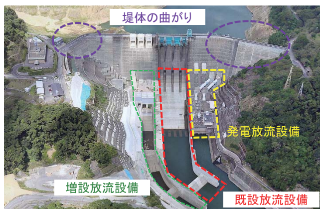
鶴田ダムの航空写真
