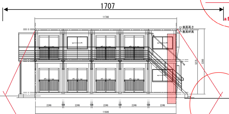
1707 通り立面図
