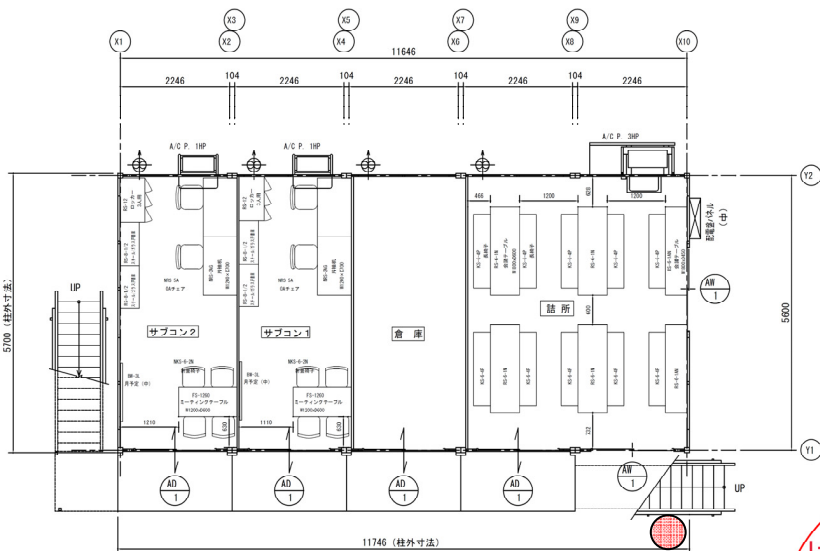
1階平面図
