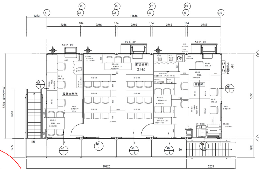
2階平面図
