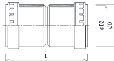
管路材(継ぎ手:ソケットタイプ) 詳細図
