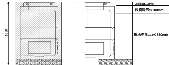
復旧断面図(MH部)
