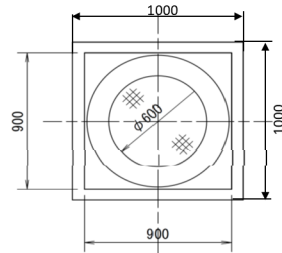
マンホール詳細図
