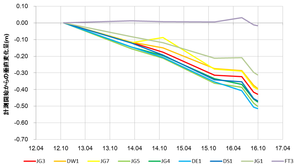
図. 6 GNSS 観測による平成新山(溶岩ドーム)の垂直変位量 (H24. 10. 24～H28. 9. 27)
