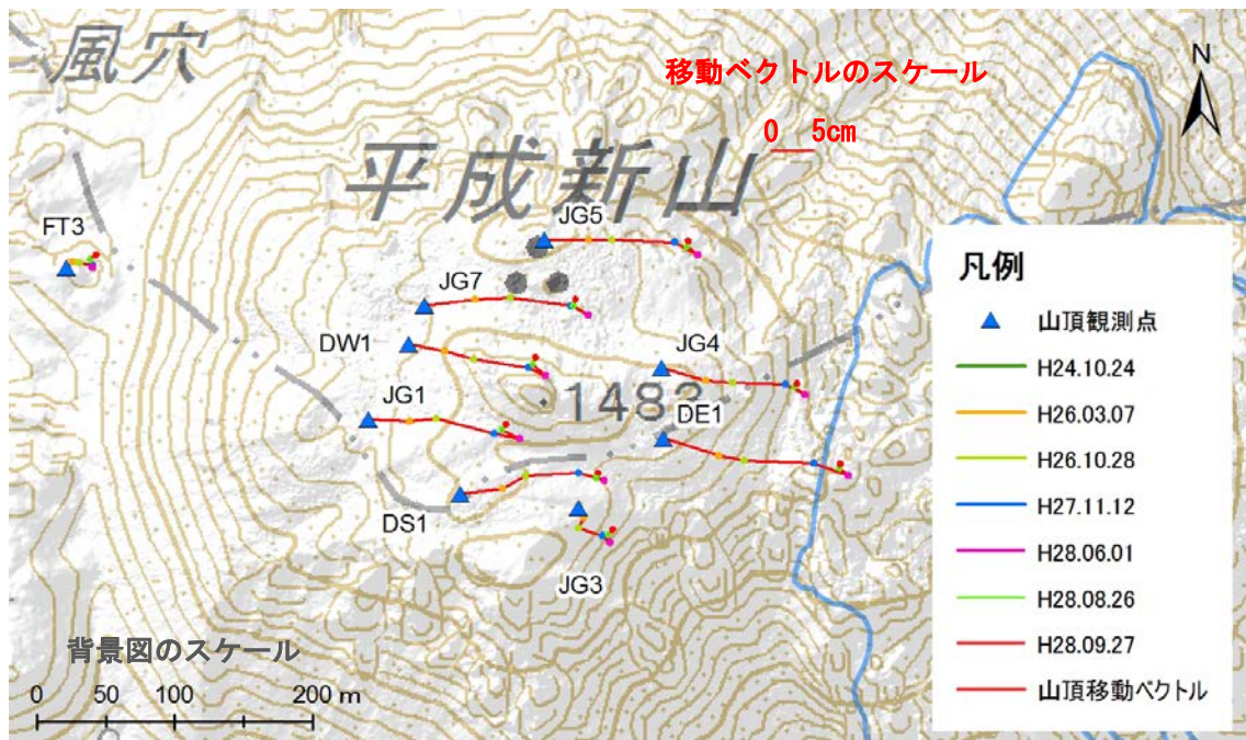
図. 5 GNSS 観測による平成新山(溶岩ドーム)の移動ベクトル (H24. 10. 24～H28. 8. 26)
