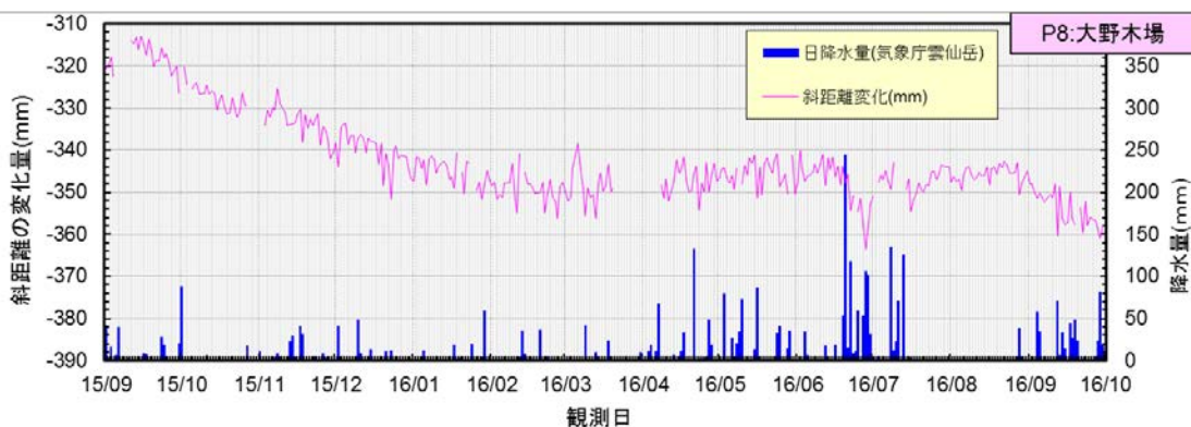
図. 1 光波測距儀の観測結果の推移
