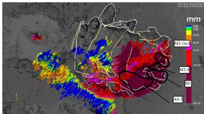
図.4 現地点での観測開始からの変化分布（平成25年6月21日～平成29年5月1日）
