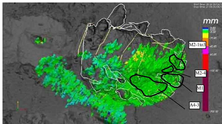
図.2 4月の変化分布（平成29年4月1日～平成29年5月1日）
