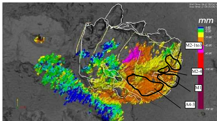
図.3 直近1年の変化分布(平成28年4月30日～平成29年5月1日)
