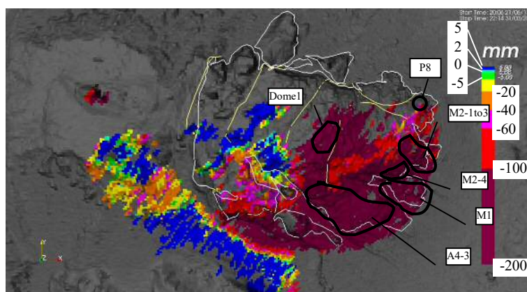
図. 4 現地点での観測開始からの変化分布（平成 25 年 6 月 21 日～令和 2 年 4 月 30 日）
