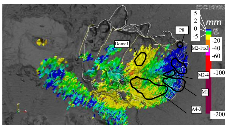
図. 3 直近 1 年の変化分布（令和元年 5 月 1 日～令和 2 年 4 月 30 日）
