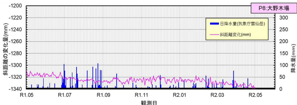
図. 2 大野木場みらい館～P8 間累計変化グラフ (H31 年 2 月～R2 年 4 月の拡大図)
