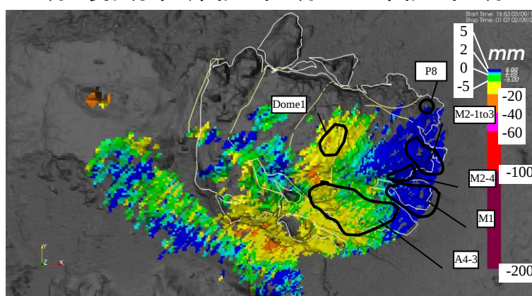
図.3 直近 1 年の変化分布（令和元年 9 月 1 日～令和 2 年 8 月 31 日）
