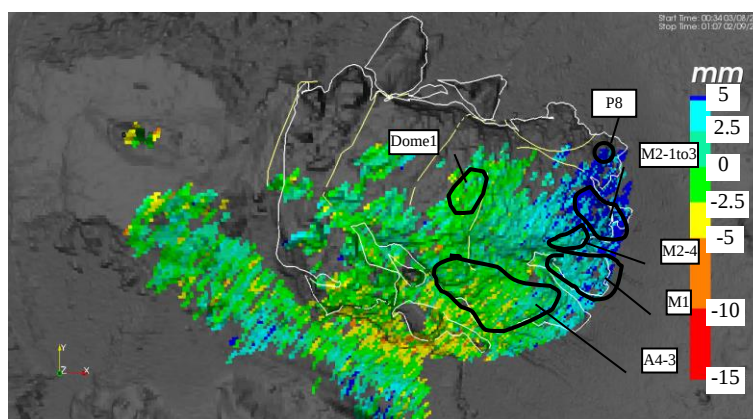
図.2 8 月の変化分布（令和 2 年 8 月 1 日～令和 2 年 8 月 31 日）
