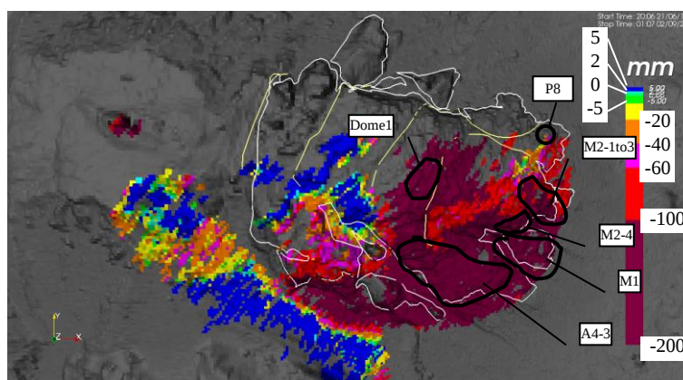
図.4 現地点での観測開始からの変化分布（平成 25 年 6 月 21 日～令和 2 年 8 月 31 日）
