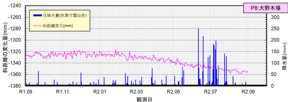
図. 2 大野木場みらい館～P8 間累計変化グラフ (R1 年 9 月～R2 年 8 月の拡大図)
