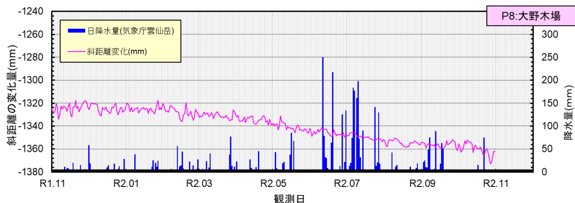
図. 2 大野木場みらい館～P8 間累計変化グラフ (R1 年 11 月～R2 年 10 月の拡大図)
