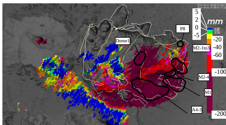
図.4 現地点での観測開始からの変化分布（平成 25 年 6 月 21 日～令和 2 年 10 月 31 日）
