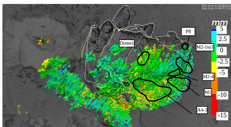
図.2 10 月の変化分布（令和 2 年 10 月 1 日～令和 2 年 10 月 31 日）
