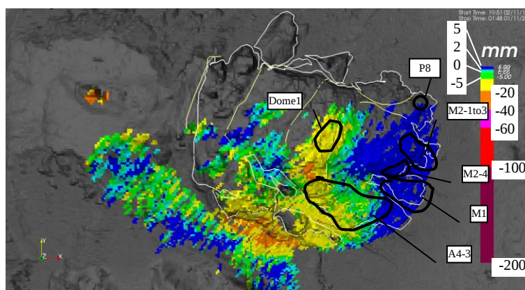
図.3 直近 1 年の変化分布（令和元年 11 月 1 日～令和 2 年 10 月 31 日）
