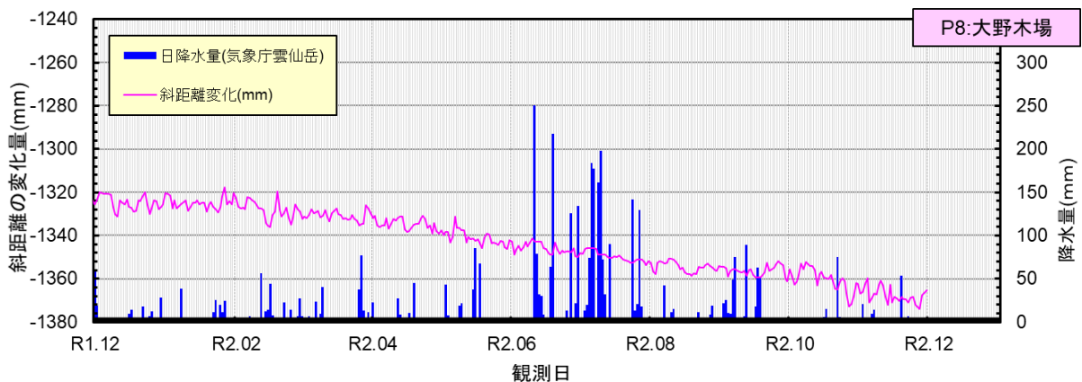
図. 2 大野木場みらい館～P8 間累計変化グラフ (R1 年 12 月～R2 年 11 月の拡大図)
