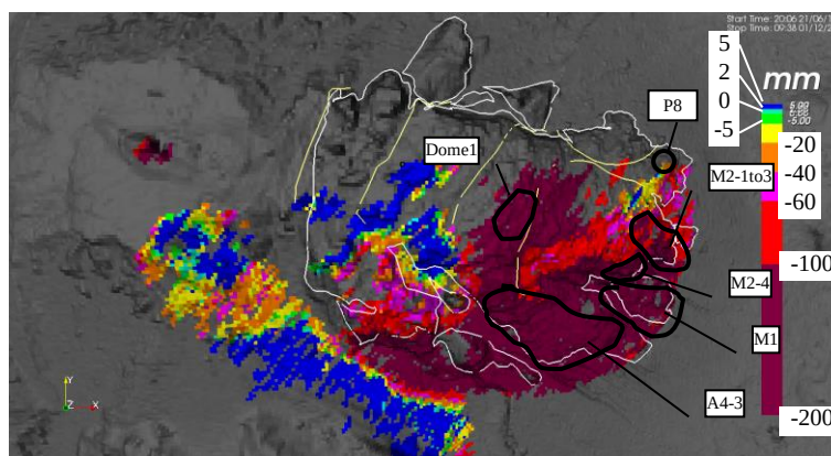
図.4 現地点での観測開始からの変化分布（平成 25 年 6 月 21 日～令和 2 年 11 月 30 日）
