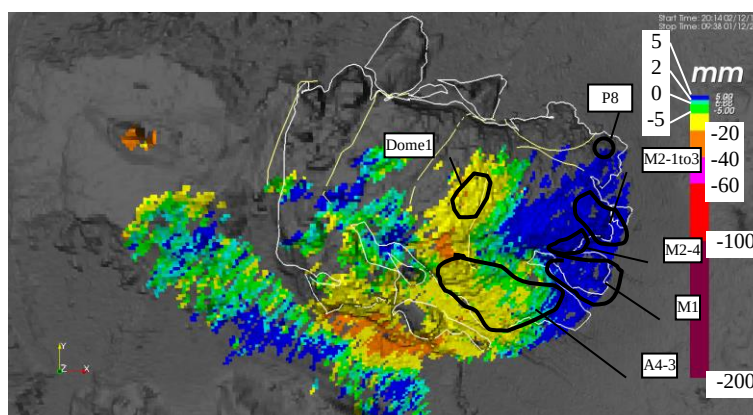
図.3 直近 1 年の変化分布（令和元年 12 月 1 日～令和 2 年 11 月 30 日）
