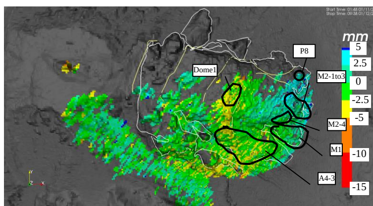
図.2 11 月の変化分布（令和 2 年 11 月 1 日～令和 2 年 11 月 30 日）
