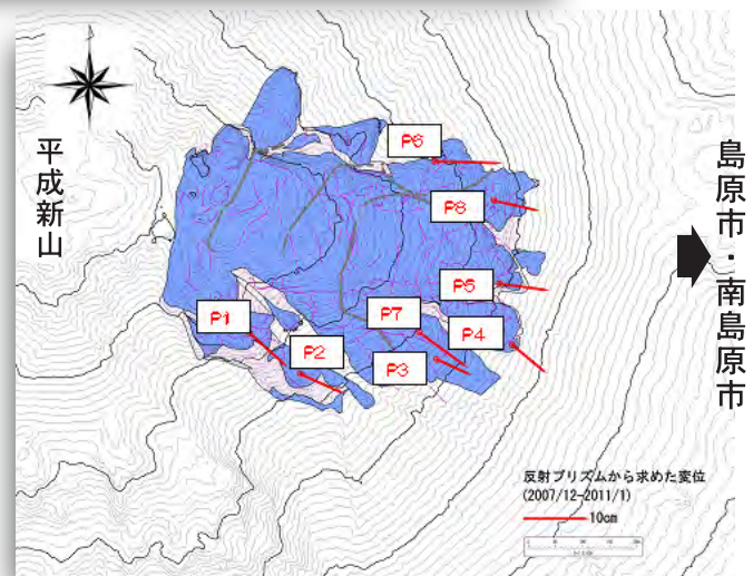
図-2 溶岩ドームの移動方向 ※平成19年12月～平成23年1月の観測データ
