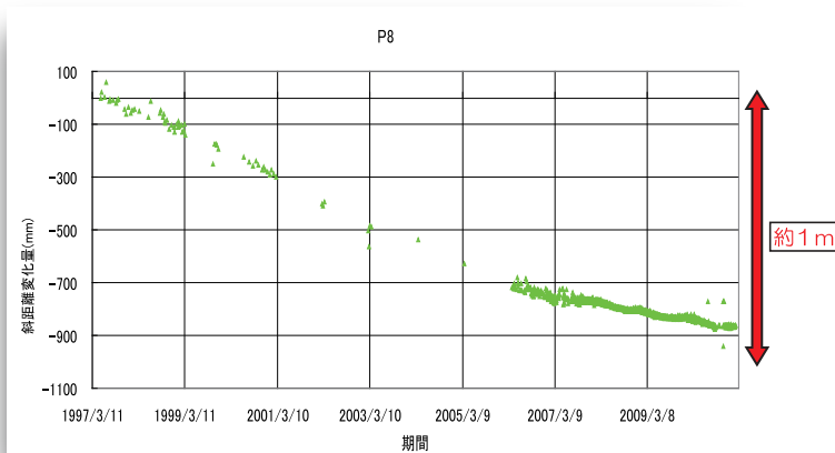
図-1 溶岩ドームの移動量 ※平成9年～平成23年の観測データ(P8)
