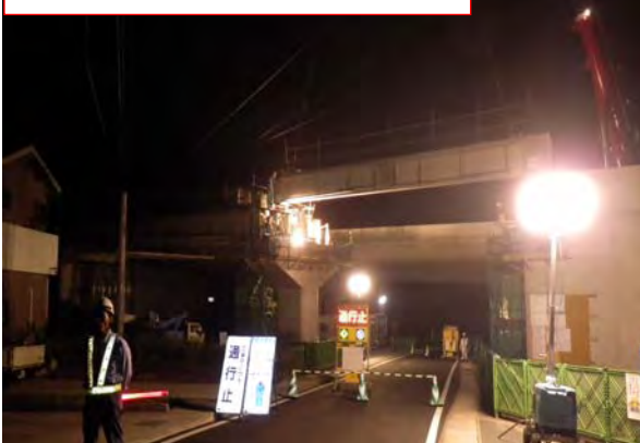
● 新湊高架橋Aランプ橋夜間架設状況
