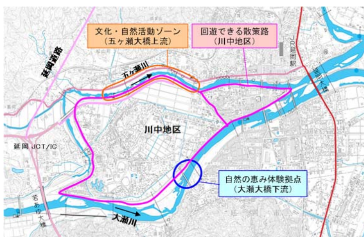
図-2 五ヶ瀬川かわまちづくり体験拠点
