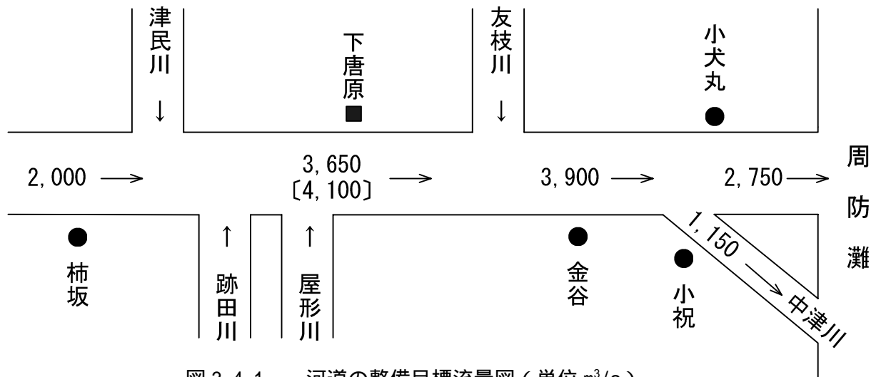
図 3.4.1 河道の整備目標流量図 (単位 m^3/s )
