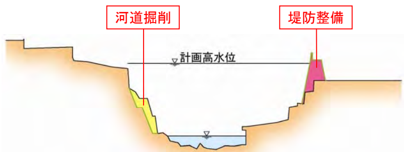
図 4. 2. 2 (2) 河道掘削及び堤防整備のイメージ（山国川 16k400 付近）
