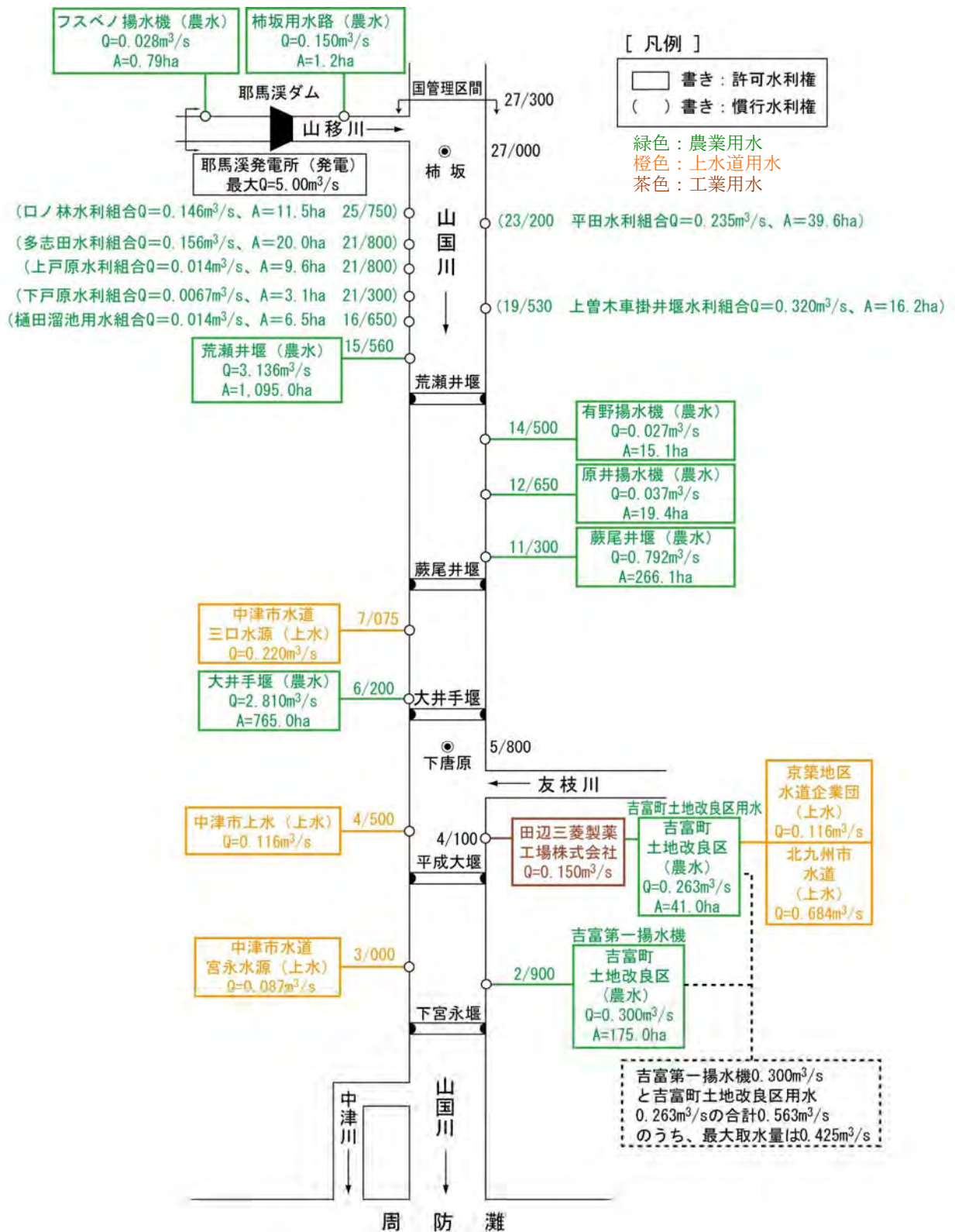
図 2.2.1 山国川水系の主な水利用の現況模式図
