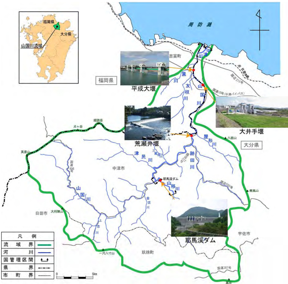
図 1. 3. 3 山国川の主な利水施設
