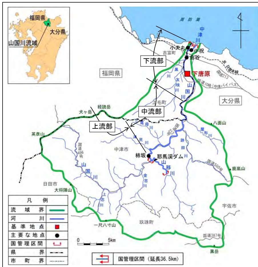
図 3.4.1 基準地点「下唐原」位置図
