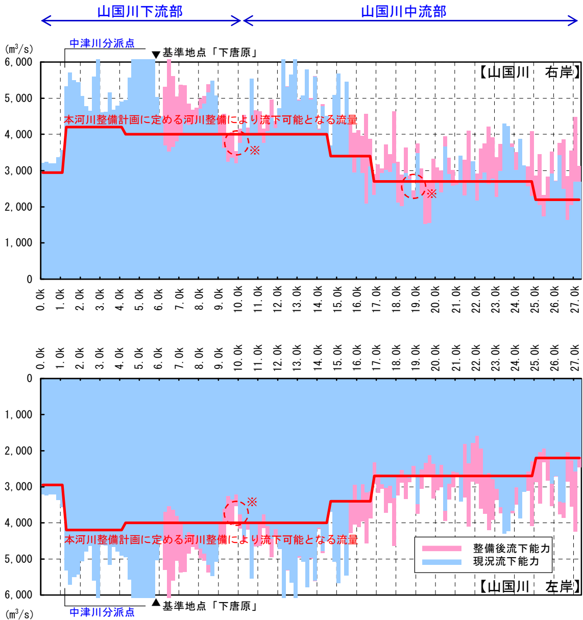
図 4. 2. 3 現況流下能力および整備後流下能力
