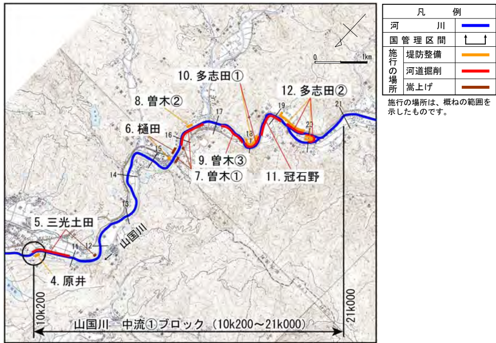
図 4. 2. 1 (2) 河道の流下能力向上対策に係る施行の場所位置図（山国川中流①ブロック）
