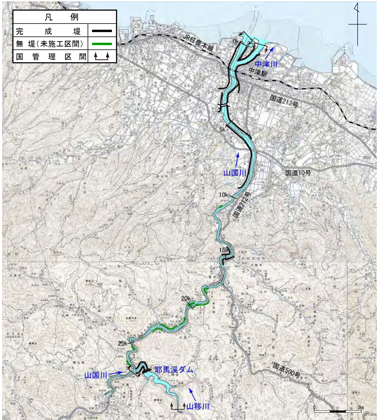
図 2.1.2 山国川の堤防整備状況図
