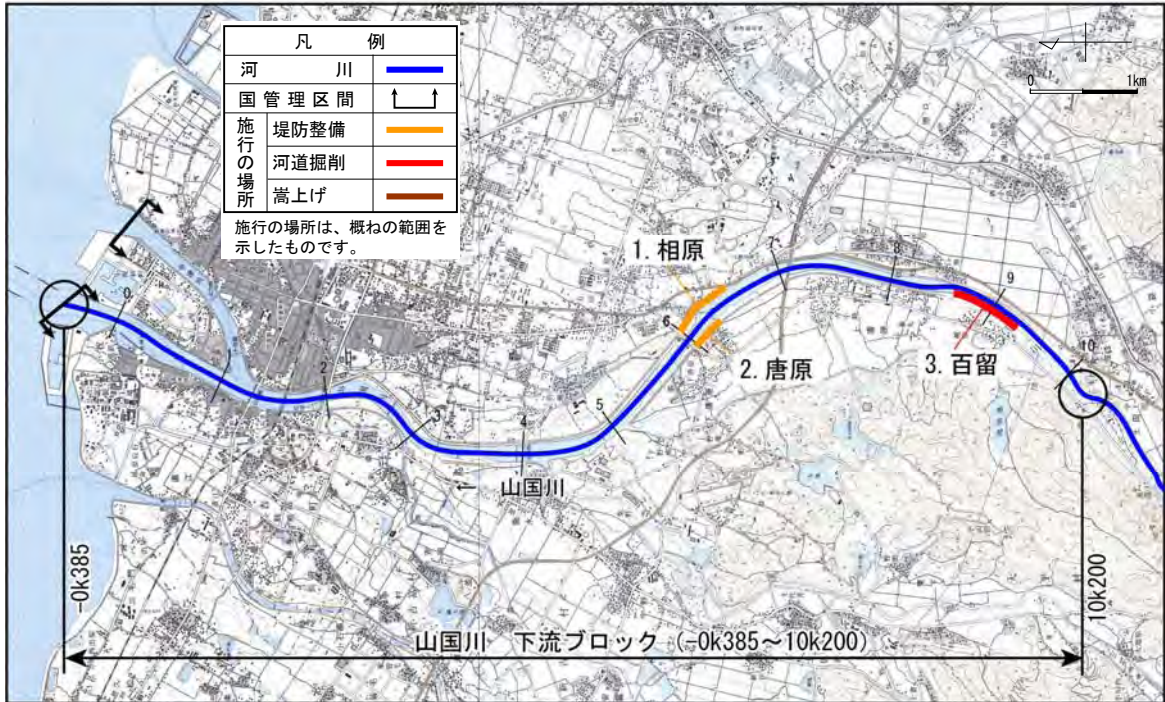
図 4. 2. 1 (1) 河道の流下能力向上対策に係る施行の場所位置図（山国川下流ブロック）
