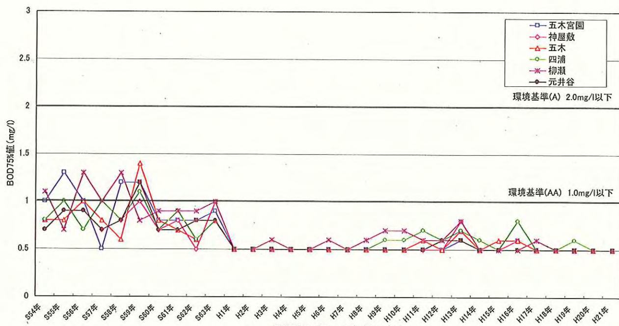
川辺川における水質の変化 図一3 水質経年変化図 (BOD75%値)
