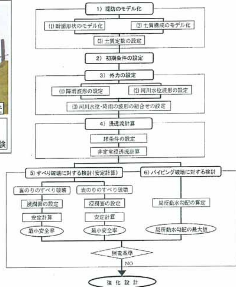
浸透に対する安全性照査の手順
