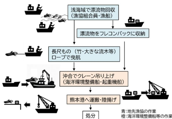
図-8 回収作業フロー図
