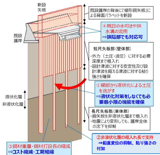
図-2 楕円鋼矢板壁工法の概要
