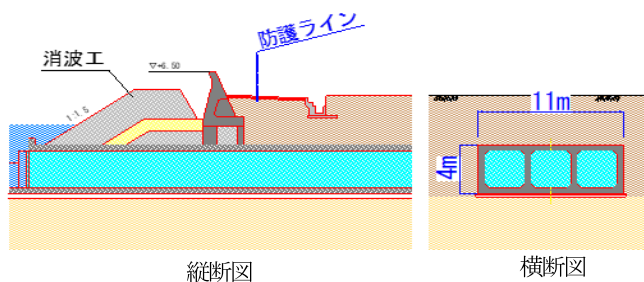
図-4 埋設管部⑥ 断面図
