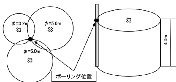
図-9 コア採取ボーリング位置図
