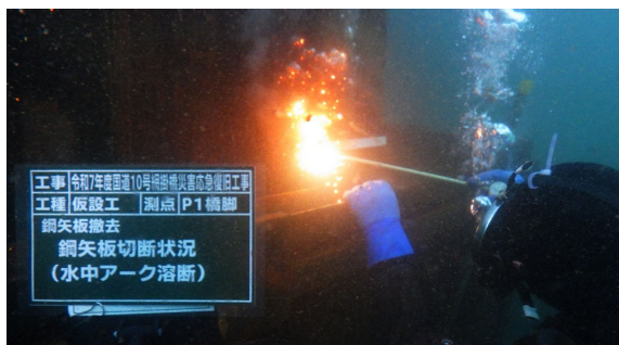
写真6 桁下施工状況
