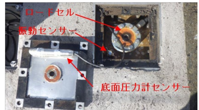
図-4 LVP センサー外観（上図）と各種センサー（下図）
