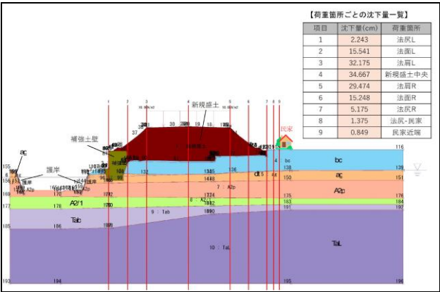
図-6 圧密沈下検討結果
