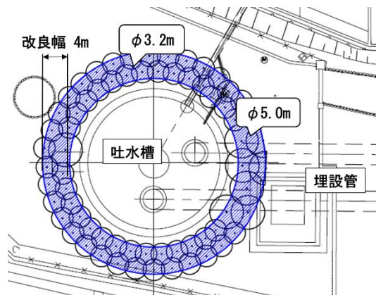
図-3 改良体配置図
