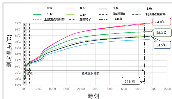
図-7 24時間経過時の温度変化
