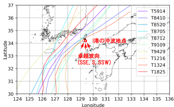
図-4 I港の沖波地点における(a)波高極値の出現頻度と分布および(b)卓越波向と選定擾乱の台風経路。
