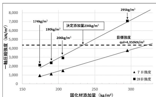
図-4 配合試験結果
