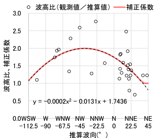
図-9 波向角と波高比，補正係数の関係（NOWPHAS玄界灘）
