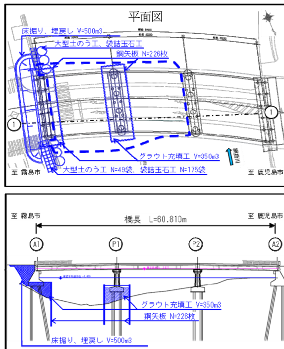
図4 応急復旧計画図
