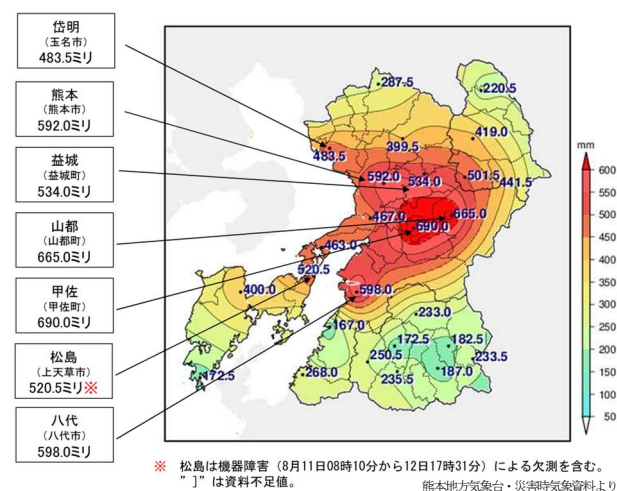
図-3 熊本県内の降水量分布
