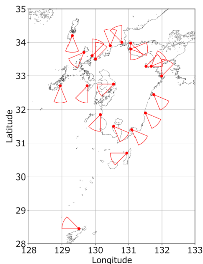
図-5 各港の沖波地点における卓越波向。扇形の波向範囲は波高極値の上位1/20平均値による卓越波向とその両隣1波向を含む3波向を意味する。
