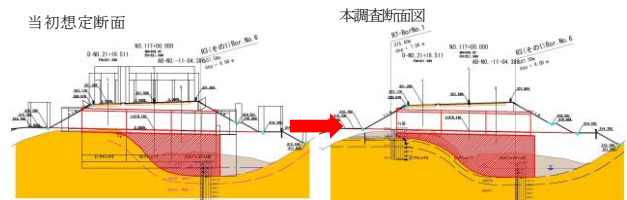
図-4 地質想定断面図
