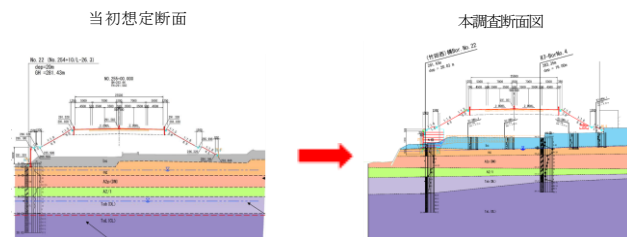
図-5 地質想定断面図
