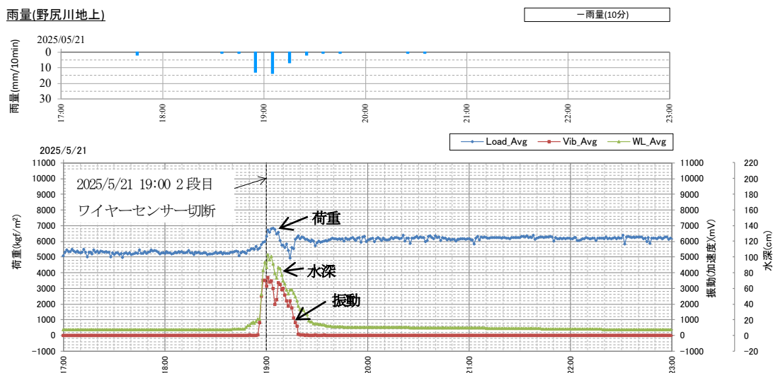
図-6 LVP センサーによる計測事例（2025 年 5 月 21 日）
