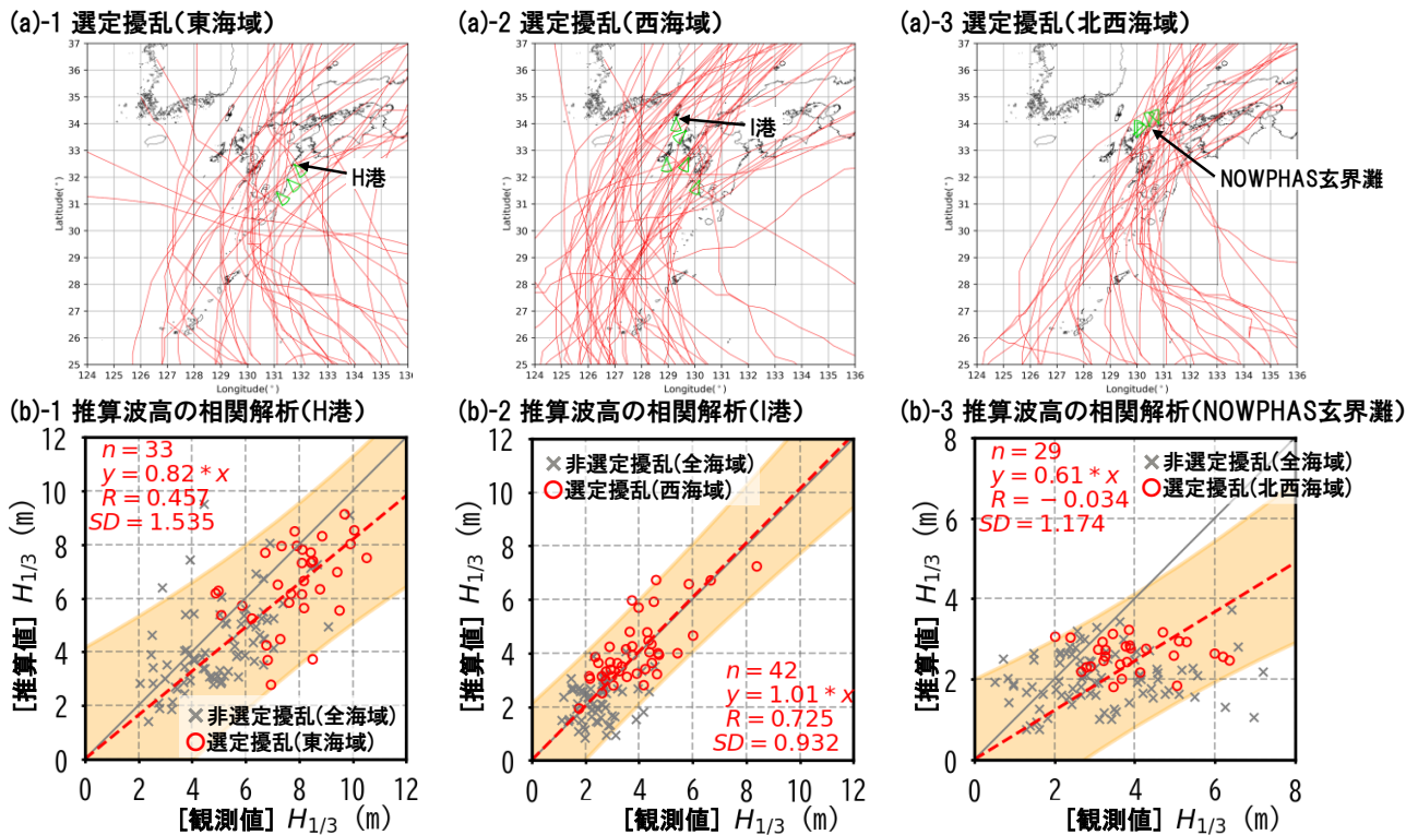
図-8 海域毎に選定した擾乱の(a)台風経路および(b)代表地点における波高極値の相関解析。(b)において赤色の○印プロットは選定擾乱の極値を、灰色の×印プロットは非選定の擾乱の極値を表す。赤字で示すnは擾乱数を、数式は赤点線で示す一次回帰式を、Rは相関係数を、SDは誤差(推算値-観測値)の標準偏差を、オレンジ色の帯は信頼度95%の予測区間を表し、全て赤色の○印プロットによる結果である。
