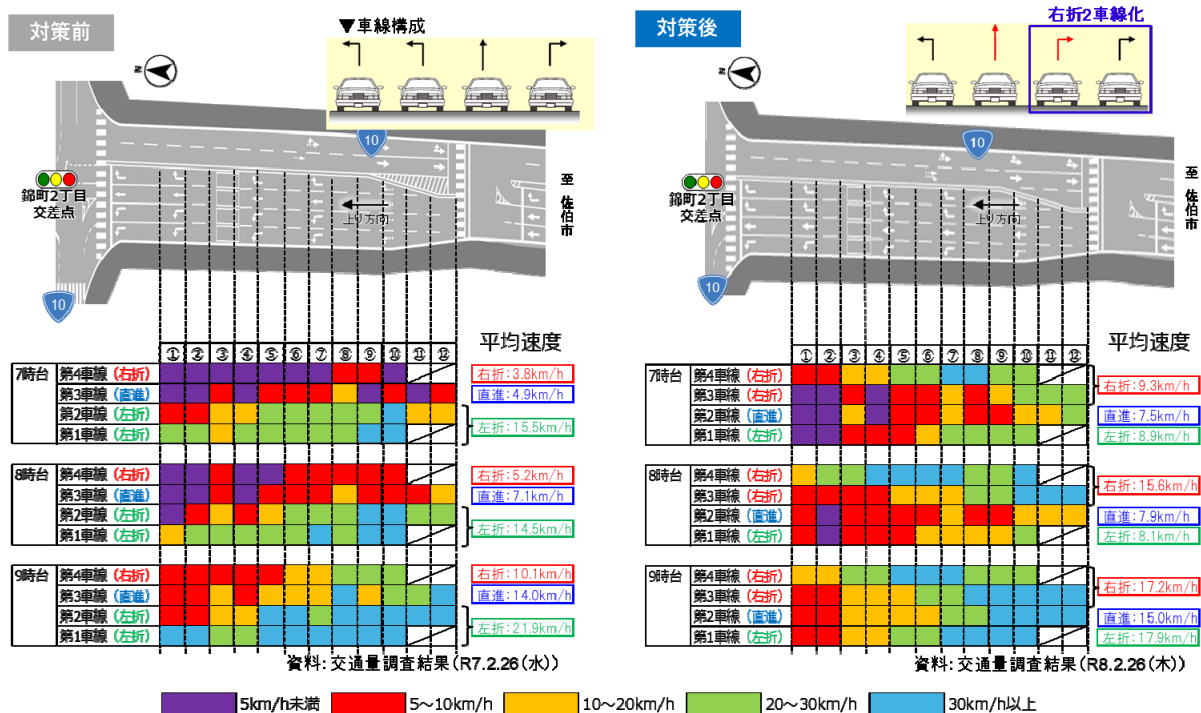
図-8 車線別時間帯別旅行速度図（10mピッチで集計）
