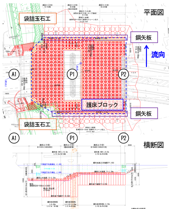
図-7 本復旧計画図
