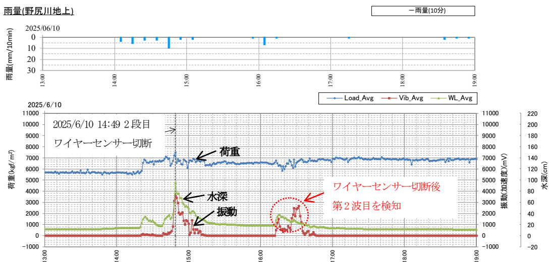
図-7 LVP センサーによる計測事例（2025 年 6 月 10 日）
