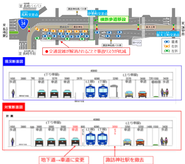
図-3 馬町交差点改良計画図(4車線化)
