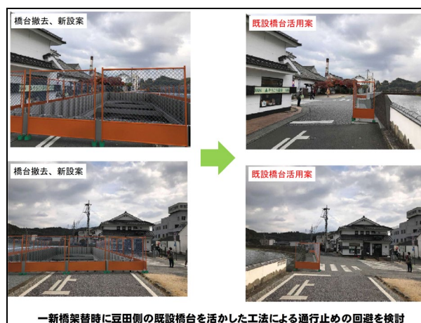
図-6 既設橋台活用案について
