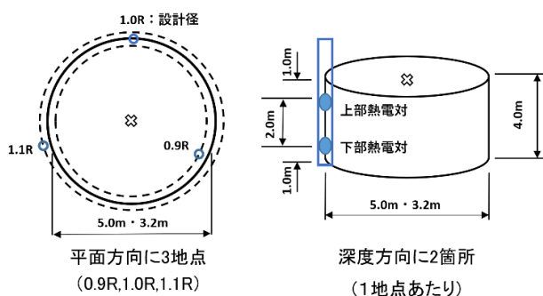
図-5 熱電対の設置位置
