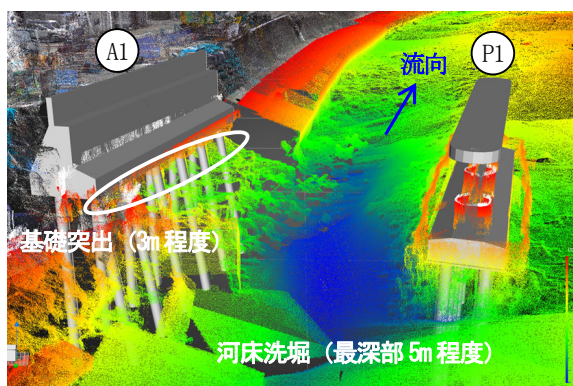
図-3 三次元化した水中ソナー調査による被災状況
