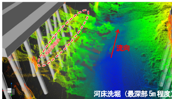
図5 水中ソナーによるがれき分布状況
