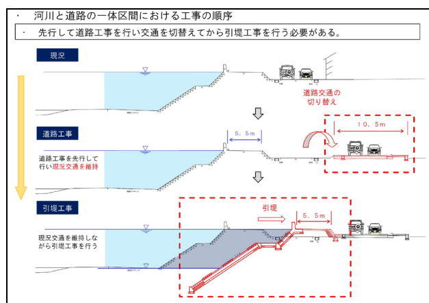
図-5 施工の手順について
