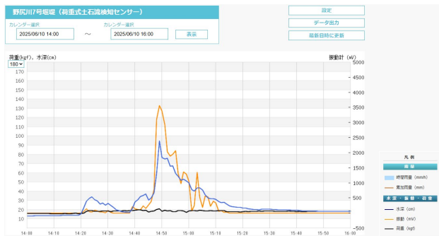
図-11 LVPセンサーシステム画面
