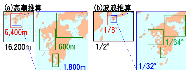
図-3 計算領域構成
