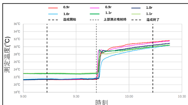
図-6 施工時の温度変化
