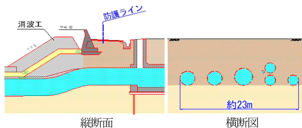
図-3 埋設管部⑤ 断面図
