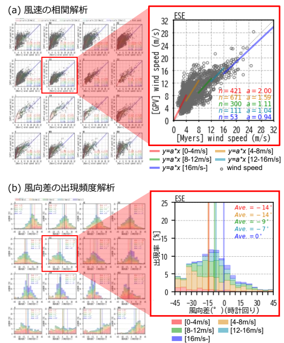
図6 16方位別・風速5ランク別の(a)風速の相関解析および(b)風向差出現頻度解析の例。(a)の回帰直線および(b)の棒グラフは風速ランク別に赤色：0～4 m/s、橙色：4～8 m/s、緑色：8～12 m/s、水色：12～16 m/s、青色：16 m/s～を意味する。
