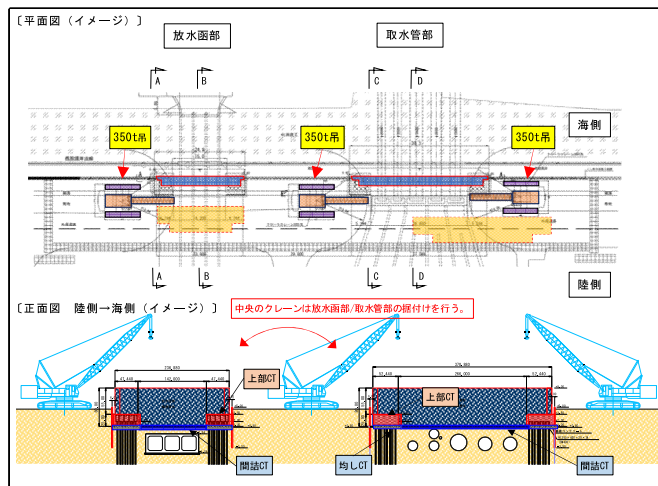
図-5 鋼製壁体の共吊り施工概要図
