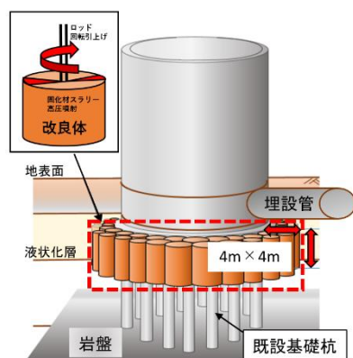
図-2 工事概要図
