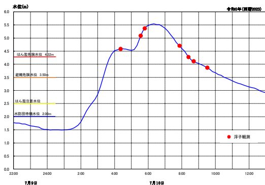
図-4 日出来橋地点 2023年浮子観測実施状況
