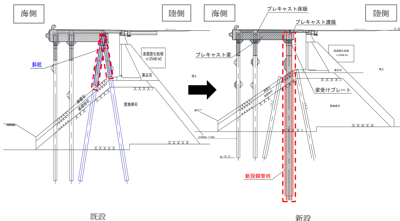
（図-1）岸壁の断面図
