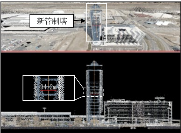
図-6 福岡空港新管制塔の高さ計測状況 （レザマップビューワによる計測）
