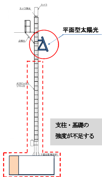
図2 シリコン系太陽光パネル設置例2
