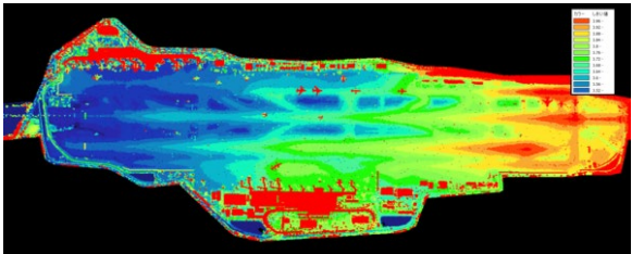
図-7 空港全域の標高分布を示すコンター図 （レザマップビューワによる作成）
