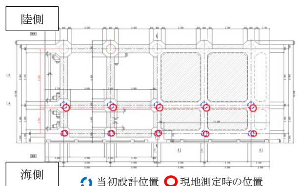
(図-5) 2次撤去工後の計測結果平面図
