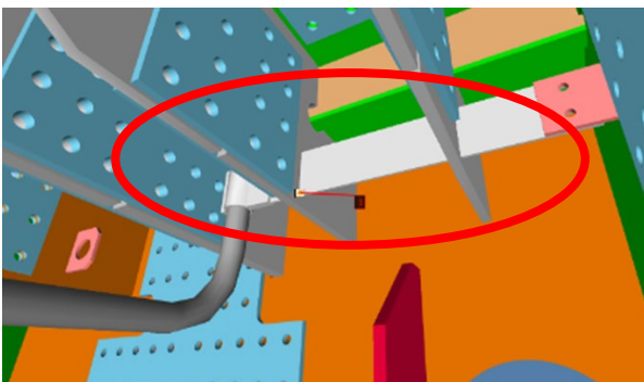
図-7 縦リブと排水支持材の干渉確認
