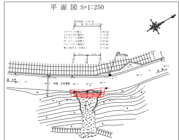
図-4 従来通り業務委託し作成された平面図
