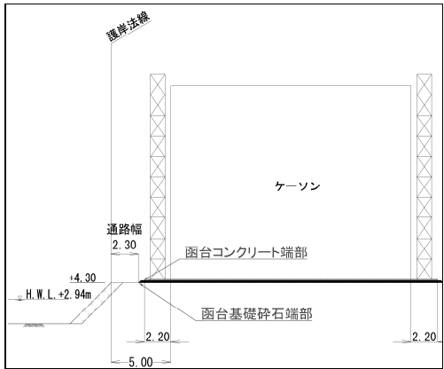
図-9 ケーソンヤード断面図
