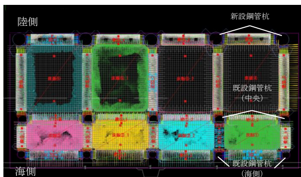
(図-6) 点群データ平面図
