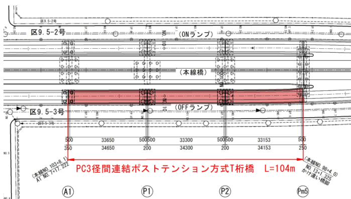
図-3 平面図
