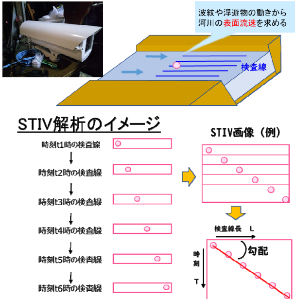
図-7 STIV手法イメージ図
