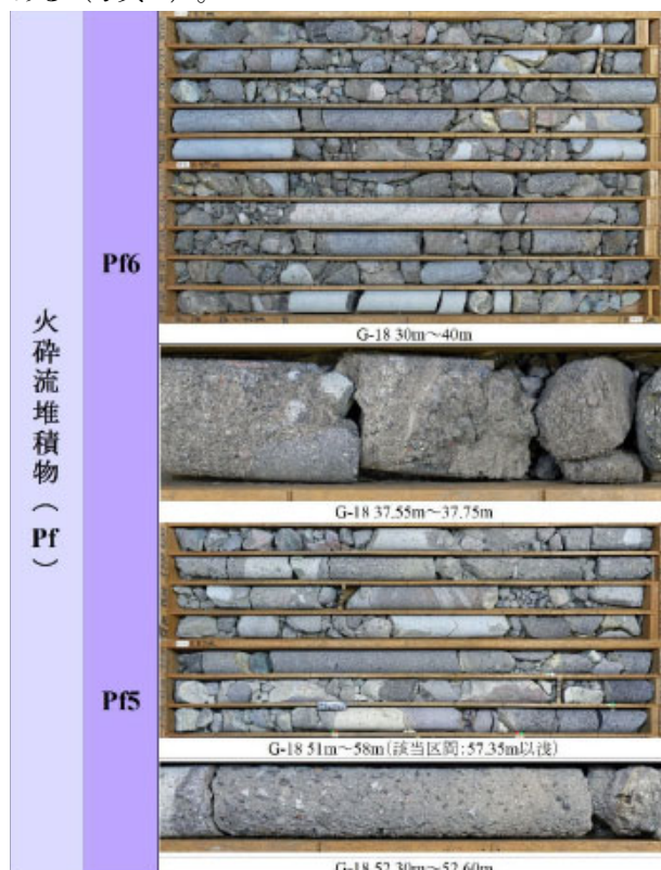
写真-1 火山性堆積物の代表コア写真
