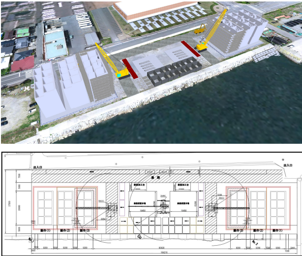
図 - 15 第4案の配置計画
