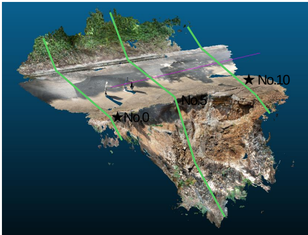
図-3 LiDARにより取得した3次元点群データ
