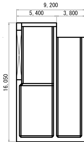
図 - 3 ケーソン断面図
