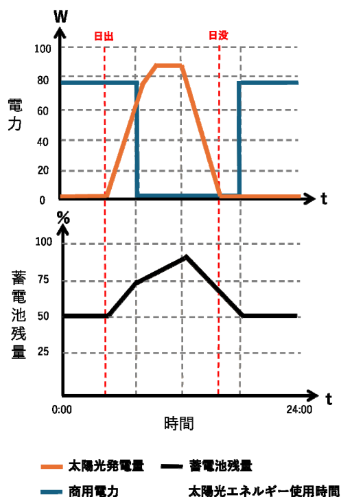
図8 蓄電池残量毎の電源切換
