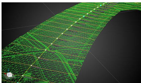
3) サーフェスモデル+線形モデル
