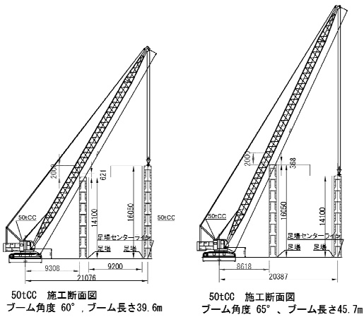
図-11 製作時のクレーン配置イメージ
