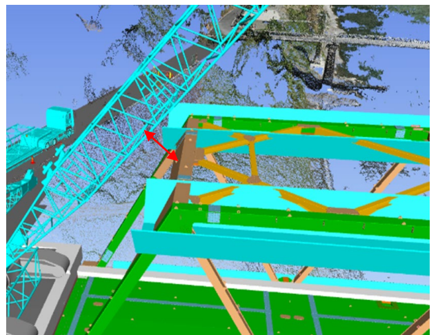
図-13 ブーム長の変更により干渉回避
