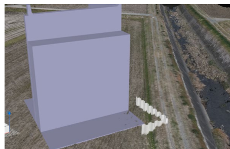
図-6 現況と3次元モデルの重ね合わせによる施工検討
