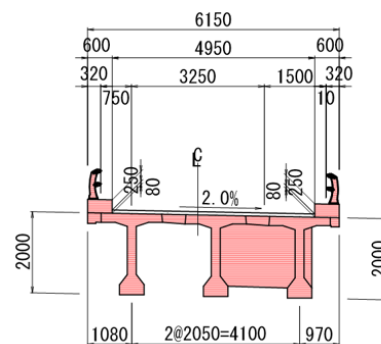
図-4 標準断面図
