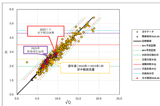
図-15 浮子観測データによる95%予測区間と非接触型流速計測法データ
