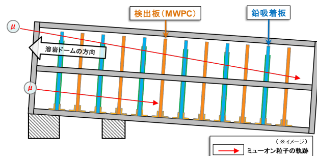
図-8 ミューオン観測器設置イメージ図
