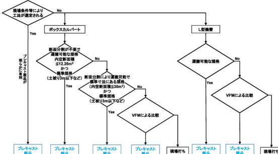
図-2 工法選定フロー（ボックスカルバート、L型擁壁）
