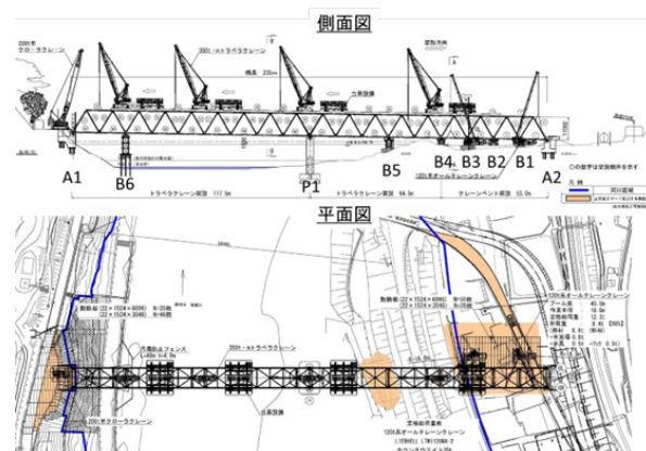
図-4 架設要領
