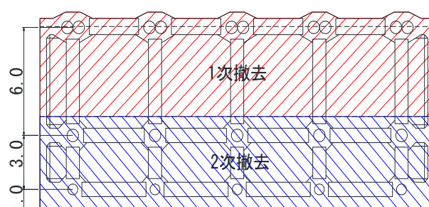
(図-3) 撤去工平面図
