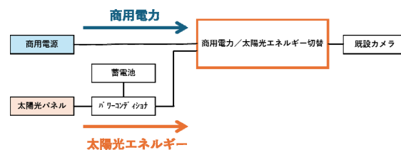
図7 商用電源・太陽光パネルの切換イメージ
