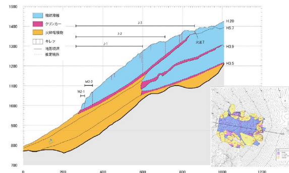
図-15 既往の検討結果における溶岩ドームの推定内部構造
