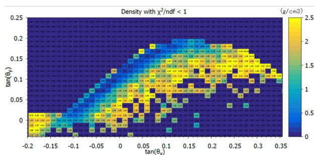
図-12 3次解析結果による密度分布図
