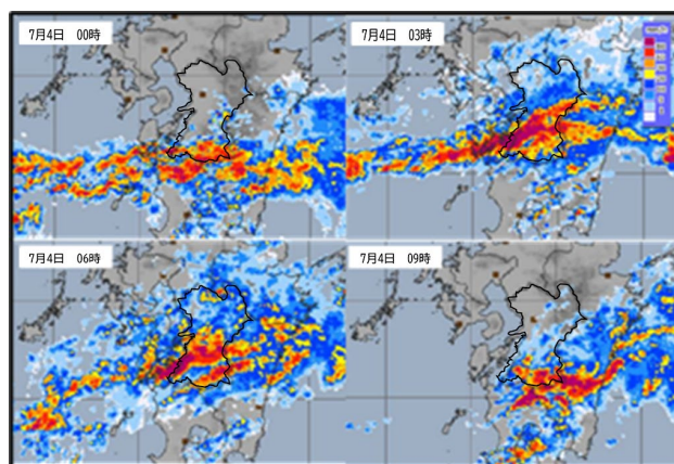
図-1 レーダー雨量 (R2.7.4 0時～9時)
