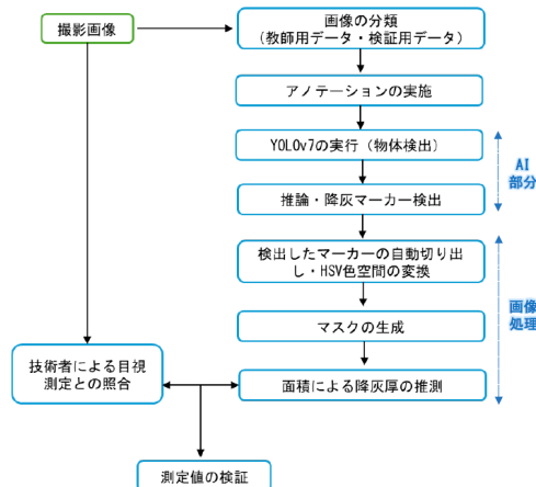
図-6 降灰厚解析手法の流れ
