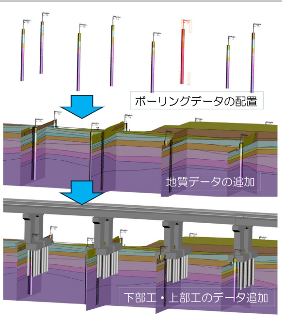
図-11 地質モデルの更新例
