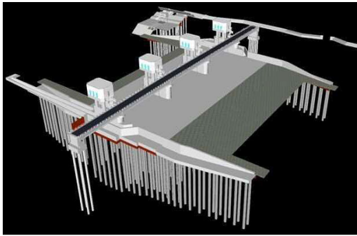
図-5 三次元モデル（新堰本体）
