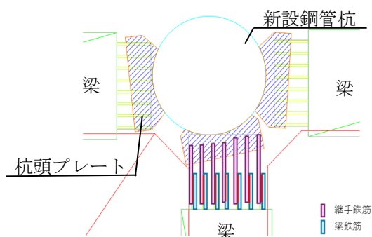
(図-7) 鉄筋継ぎ足し平面図
