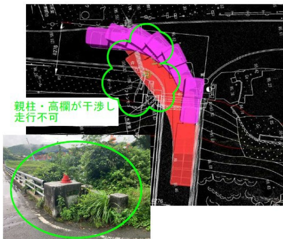
図-11 左折進入 親柱に干渉
