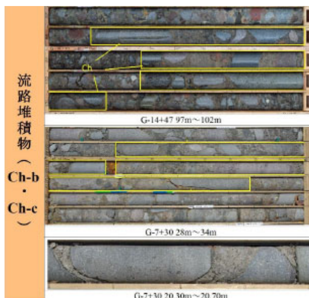
写真-2 非火山性堆積物の代表コア写真
