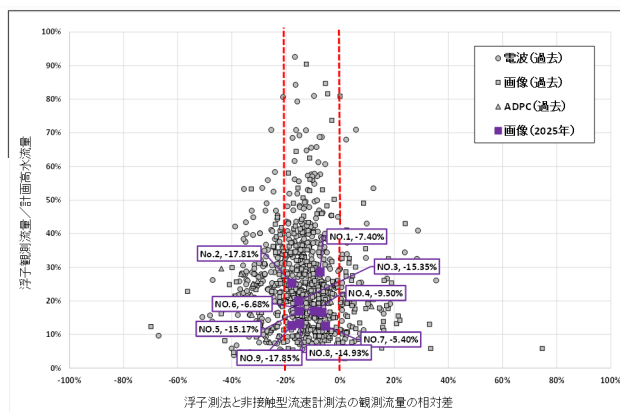
図-14 浮子とSTIV法による観測流量の相対差
