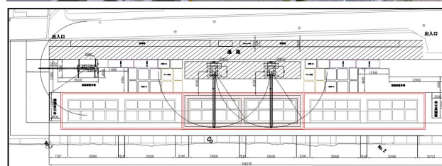
図 - 14 第3案の配置計画
