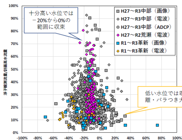
図-12 浮子と次世代の観測流量の相対差
