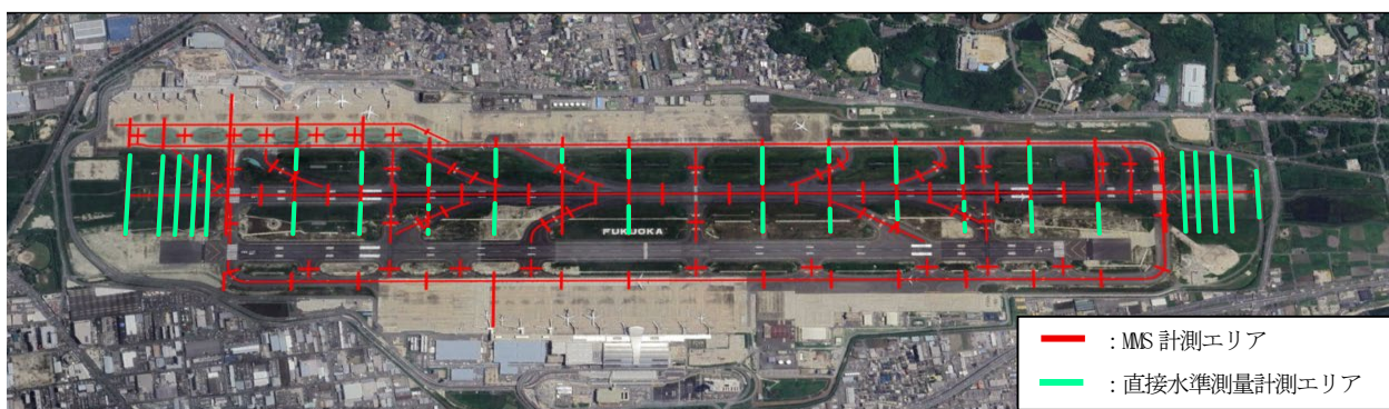
図-1 計測位置図（定期点検測量）
