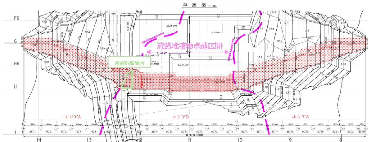
図-4 グラウチング平面図
