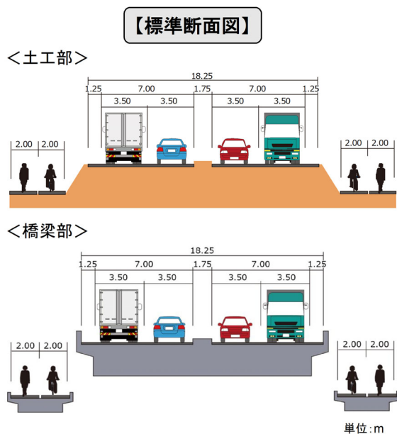
図-4 標準横断図
