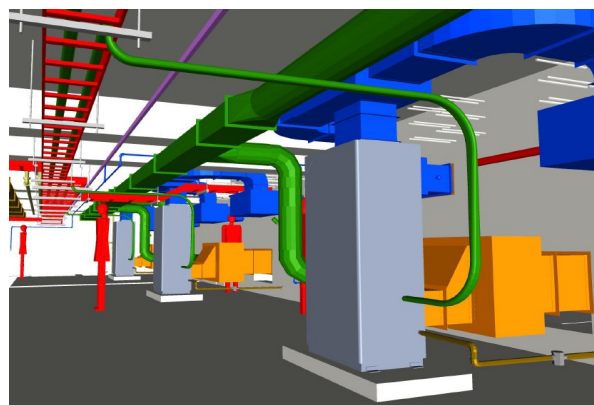
図-8 検査場BIMモデル 地下ピットの干渉チェック
