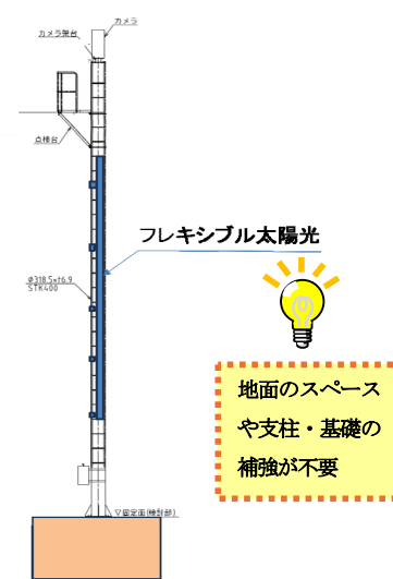
図3 薄型カルコパイライト設置例
