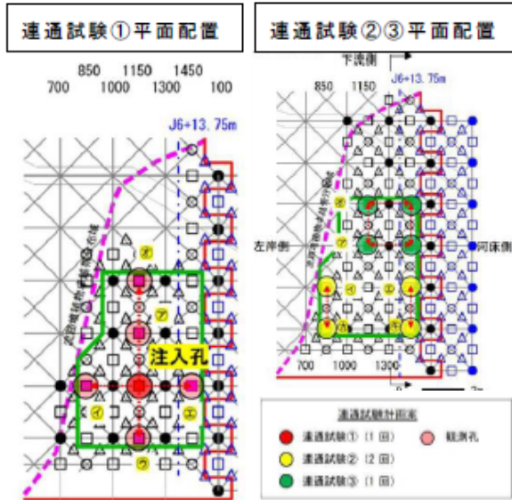
図-5 連通試験 孔配置図
