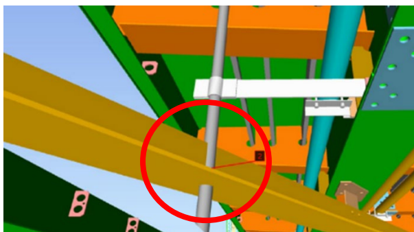
図-6 下横構とスラブドレーンの干渉確認
