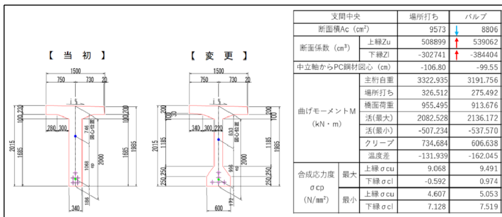
図-8 バルブ形状変更による断面性能の向上
