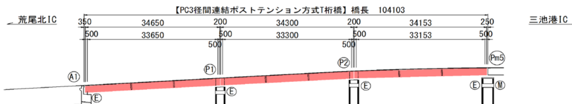
図-5 側面図
