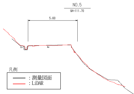
図-5 重ね合わせた横断面図
