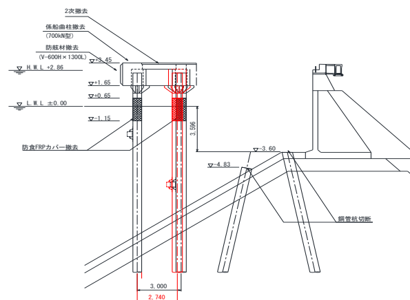
(図-4) 1次撤去工後の計測結果
