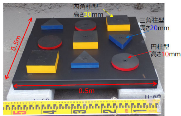
図5 降灰マーカー(凸型)
