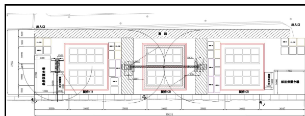
図 - 13 第2案の配置計画
