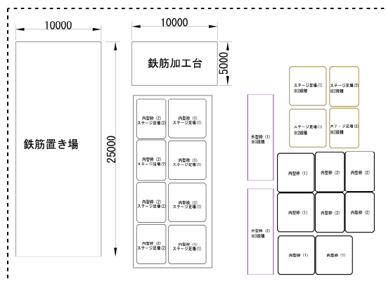
図 - 8 各資材置き場イメージ
