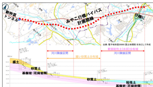
図-5 みやこ行橋バイパス付近の地質状況概念図
