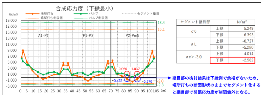
図-7 合成応力度比較
