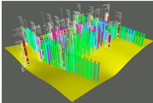
図-6 杭長の設定（地盤モデル）
