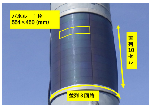
図6 フレキシブル型太陽光パネル（薄型カルコパイライト）
