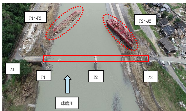
写真-2 旧相良橋被災状況
