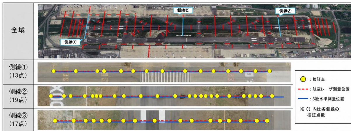
図4 精度比較検証箇所
