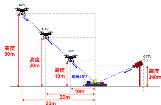
図-8 CCTVカメラ及びUAVによる撮影条件
