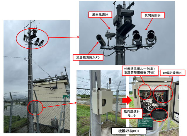
図-9 日出来橋の流量観測機器
