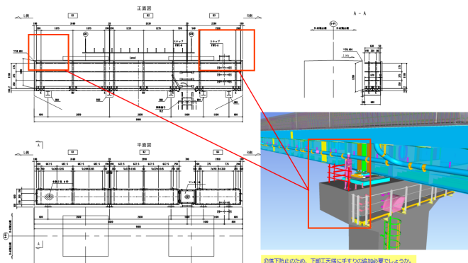
図-4 維持管理を見据えた設計照査
