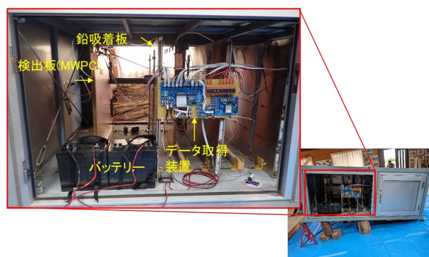
図-9 ミューオン観測器の設置状況
