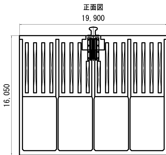
図 - 4 ケーソン正面図
