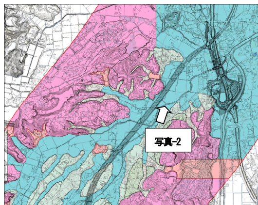
図-8 地形解析から推定される地質(平坦地部)
