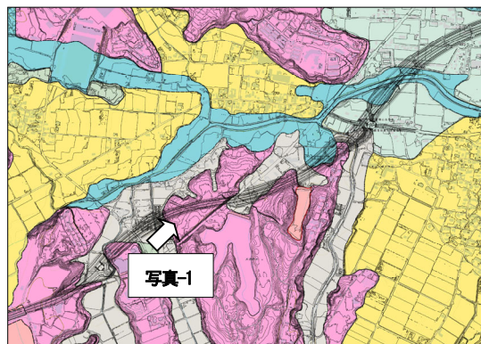
図-7 地形解析から推定される地質(山地部)
