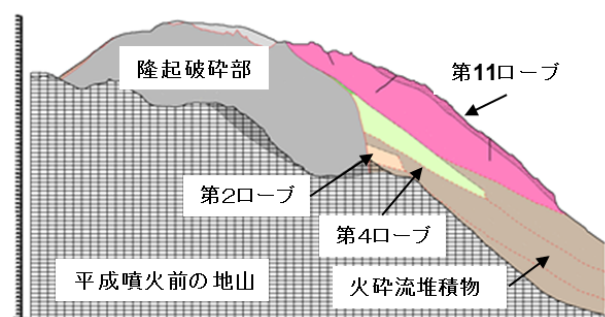
図-4 推定内部構造図(2011年の検討成果例)
