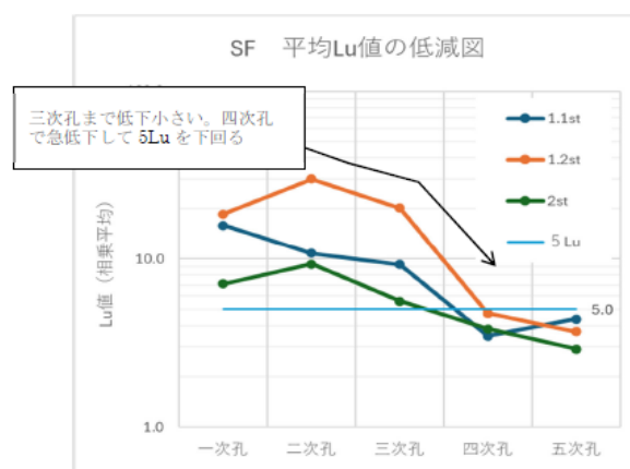
図-3 超微粒子セメント(SF)のルジオン値低減図
