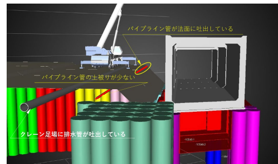
図-2 埋設物の位置・深さの設計照査
