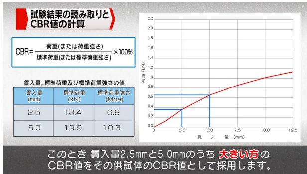
図 6 動画内 CBR 値の計算
