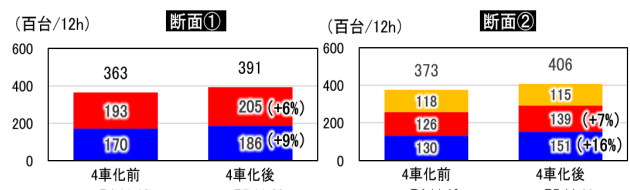
図-2 交通量推移の各断面
