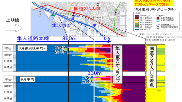
図-20 隼人東IC周辺詳細旅行速度図
