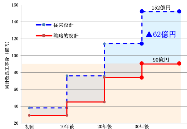
図-12 従来設計と本設計におけるLCC比較
