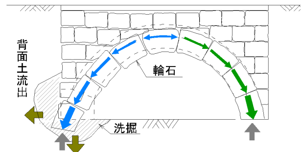
図-3 変状の事例（イメージ）
