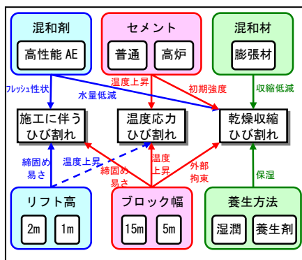
図-10 ひび割れ発生原因と対策効果の因果関係
