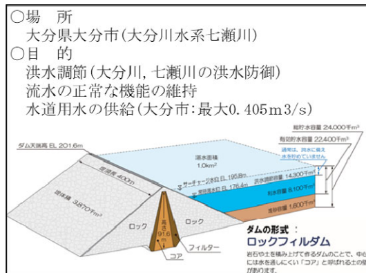
図-1 ななせダムの概要
