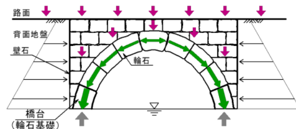
図-1 石造アーチ橋の荷重伝達経路の概念図
