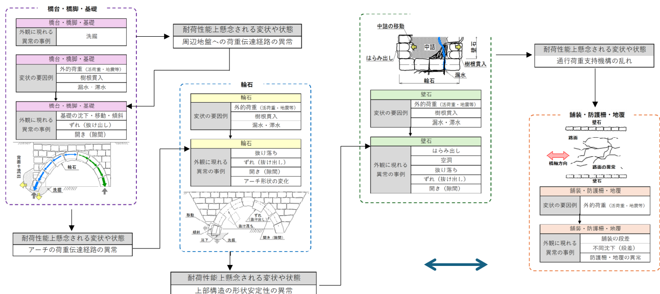
図-5 石造アーチ橋の形状変化に関する損傷とその関連性
