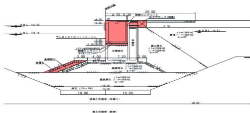
図-5 a)スリットケーソン一部取替案
