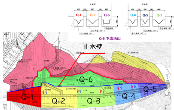
図-6 浸透量計測施設（止水壁，分水壁）配置系統図
