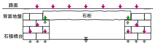
図-2 石桁橋の荷重伝達経路の概念図
