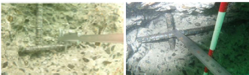
写真-4 はつり調査
