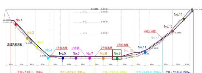
図-7 浸透流観測孔位置図
