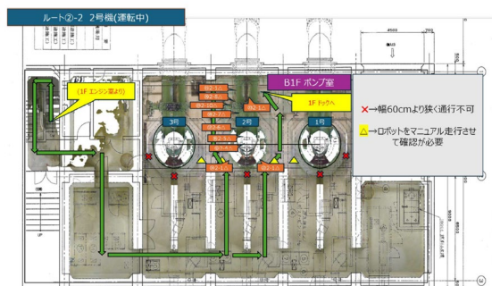
図-7 点検ルート (B1Fポンプ室)
