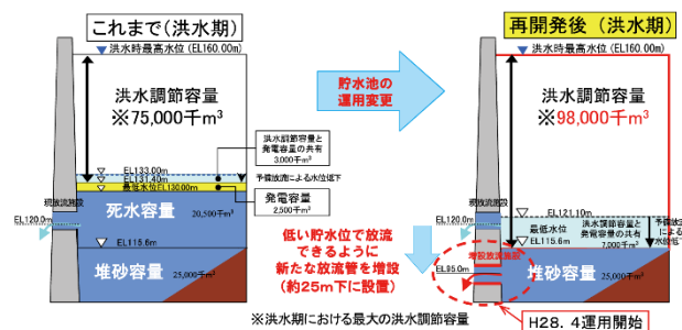
図-2 鶴田ダム再開発事業による容量配分見直し
