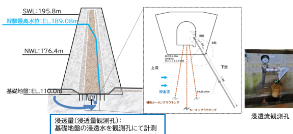
図-8 浸透量計測イメージ図（浸透流観測孔）
