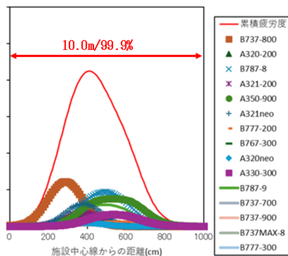
図-4 横断方向における累積疲労度分布図
