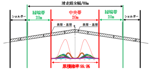
図-5 航空機主脚の走行分布と滑走路横断区分の関係
