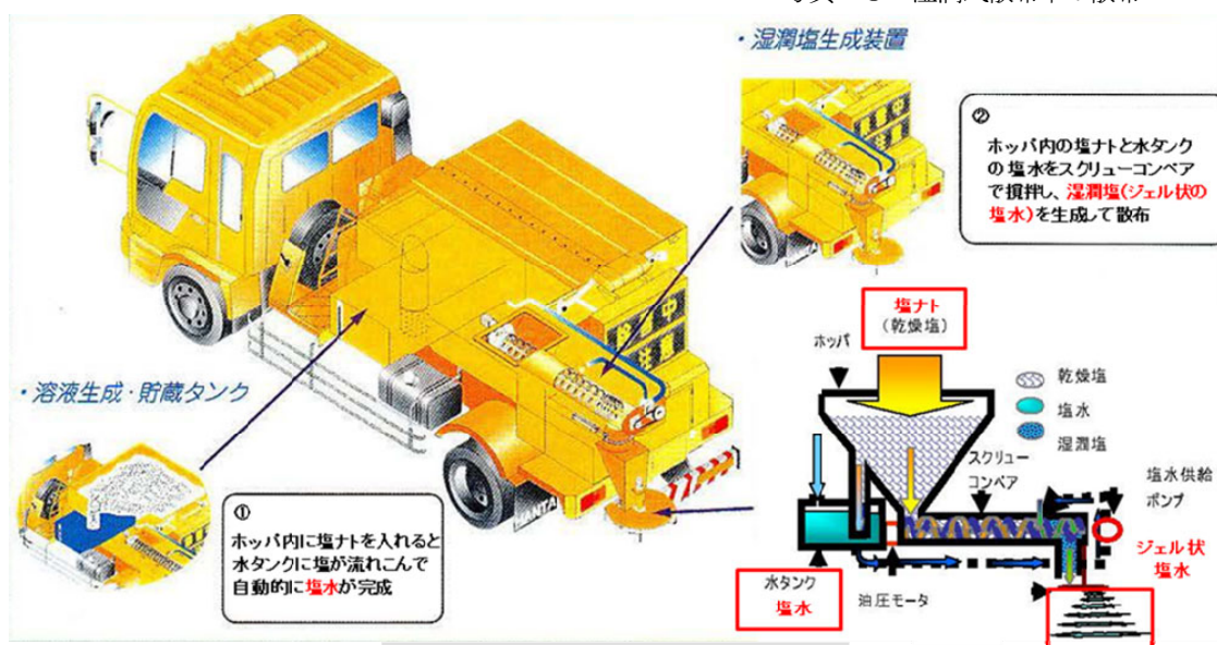
図－6 湿潤式散布車概要
