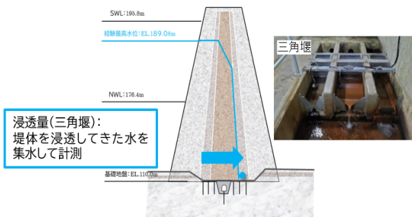
図-5 浸透量計測イメージ図（三角堰）
