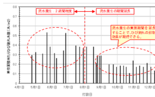
図-13 流水養生の期間延長の効果
