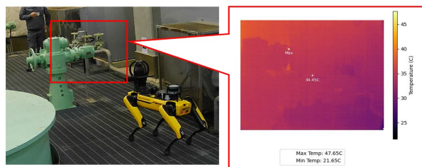
図-13 異常過熱の撮影状況
