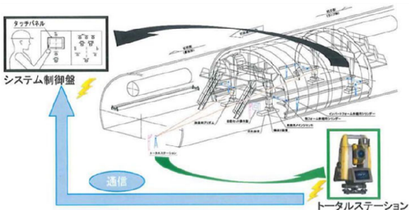
図-8 セントル自動化概要図
