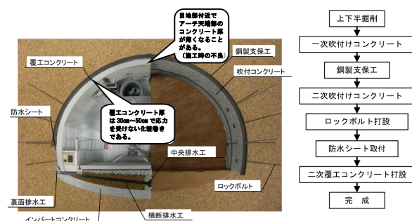
図-2 NATM工法の施工手順
