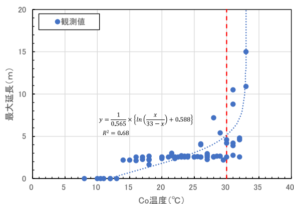
図-14 コンクリート打込み温度とひび割れの関係
