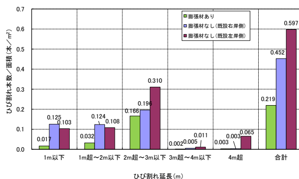
図-12 ひび割れ延長（膨張材の有無による影響）
