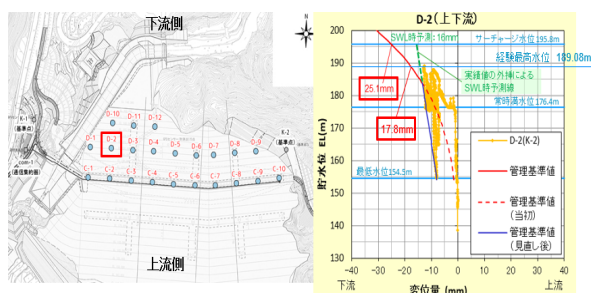
図-9 水平変位量グラフ（D-2地点）
