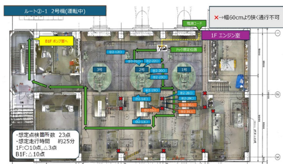
図-6 点検ルート (1Fエンジン室)
