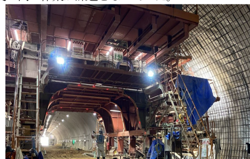
写真-4 移動式の鋼製型枠(スライドセントル)
