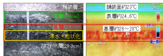
図-1 粒状化状況および赤外線画像による温度分布
