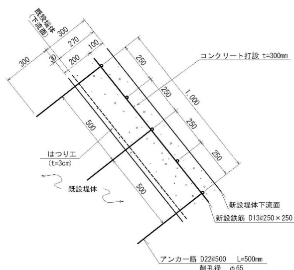
図-5 壁面補修工の基本仕様（非越流部断面）
