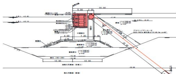
図-7 c)直立消波ブロック案
