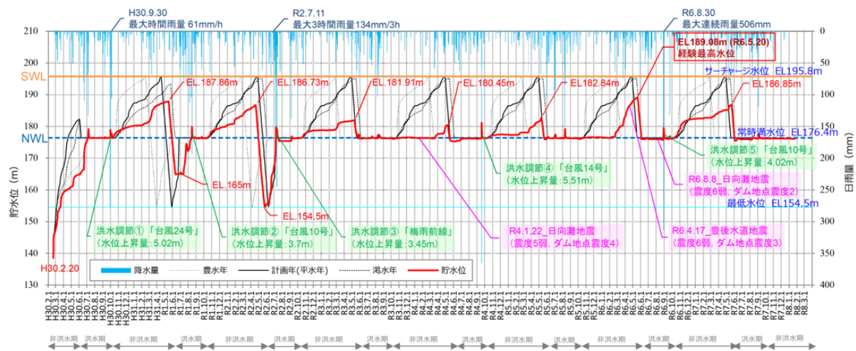
図-3 試験湛水経過図
