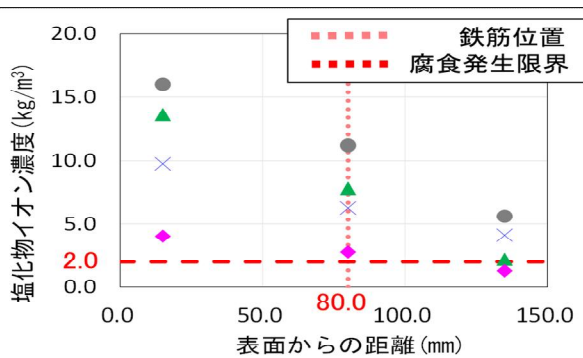
図-3 塩分含有量
