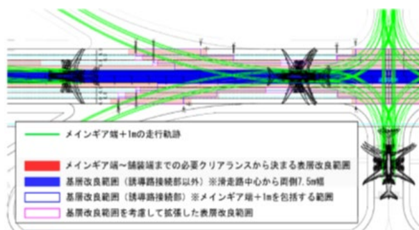
図-10 航空機走行軌跡に基づく表層・基層改良範囲の設定
