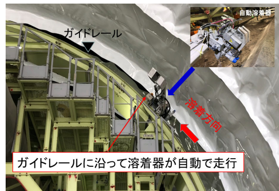
写真-3 自走式溶着器
