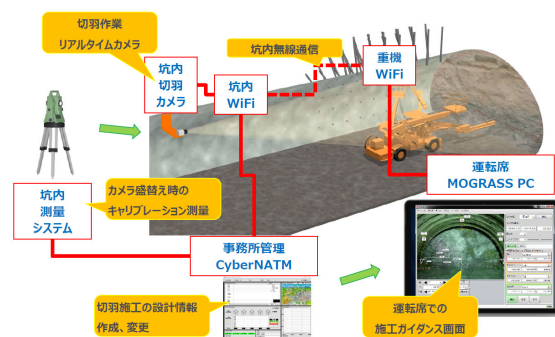
図-4 穿孔誘導システム構成図
