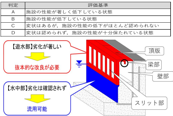
図-4 改良方針イメージ図
