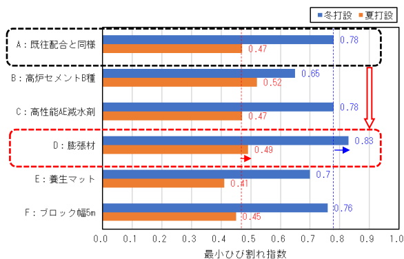
図-11 温度応力解析結果
