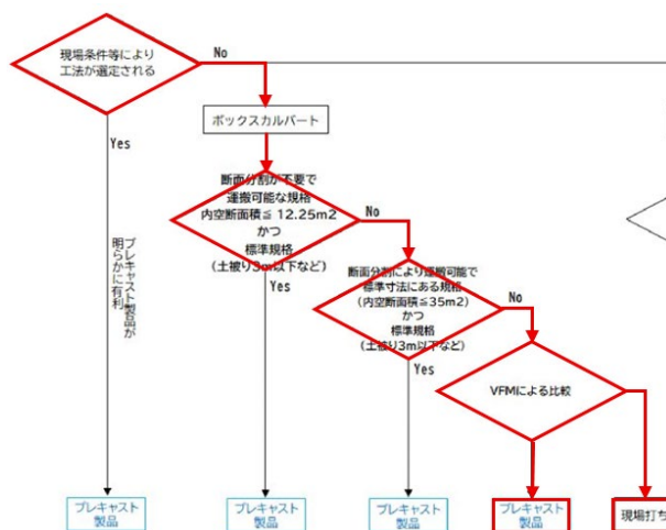
図-6 工法選定フロー[14号函渠]
