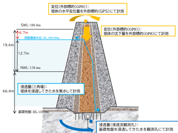
図4 堤体・基礎地盤における計測項目
