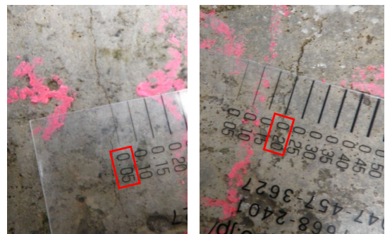
図-9 ひび割れの発生状況写真
