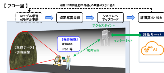
図-5 AI切羽画像評価システム
