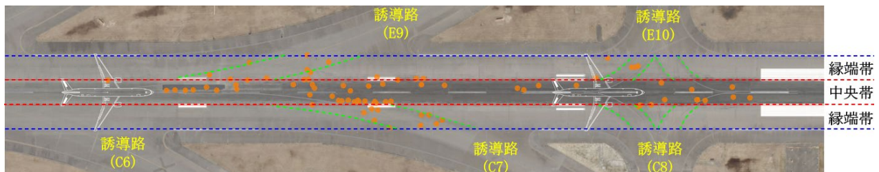
図-2 2022-2025年度における緊急補修位置の分布 (●: 補修箇所)
