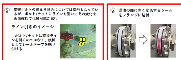
図-11 ボルトの緩みと油漏れの確認
