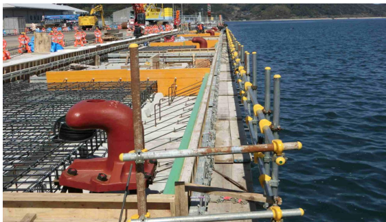
写真-10 上部工
