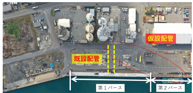
写真-11 仮設配管
