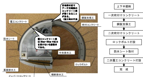
図-2 NATM工法の施工手順
