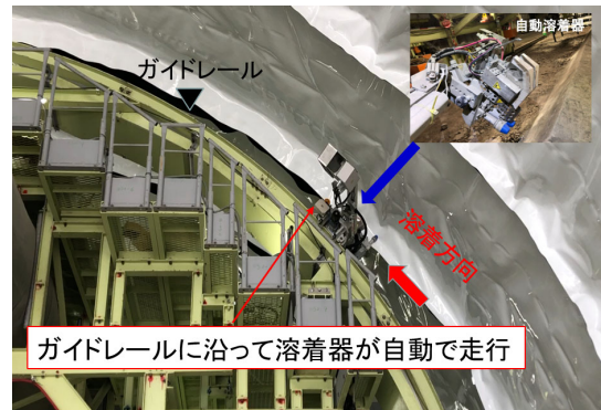
写真-3 自走式溶着器
