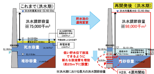
図-2 鶴田ダム再開発事業による容量配分見直し
