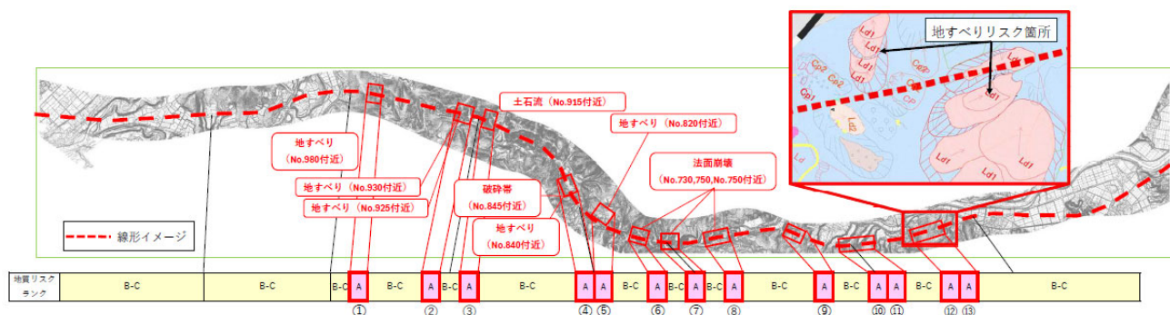
図-5 地質リスク図
